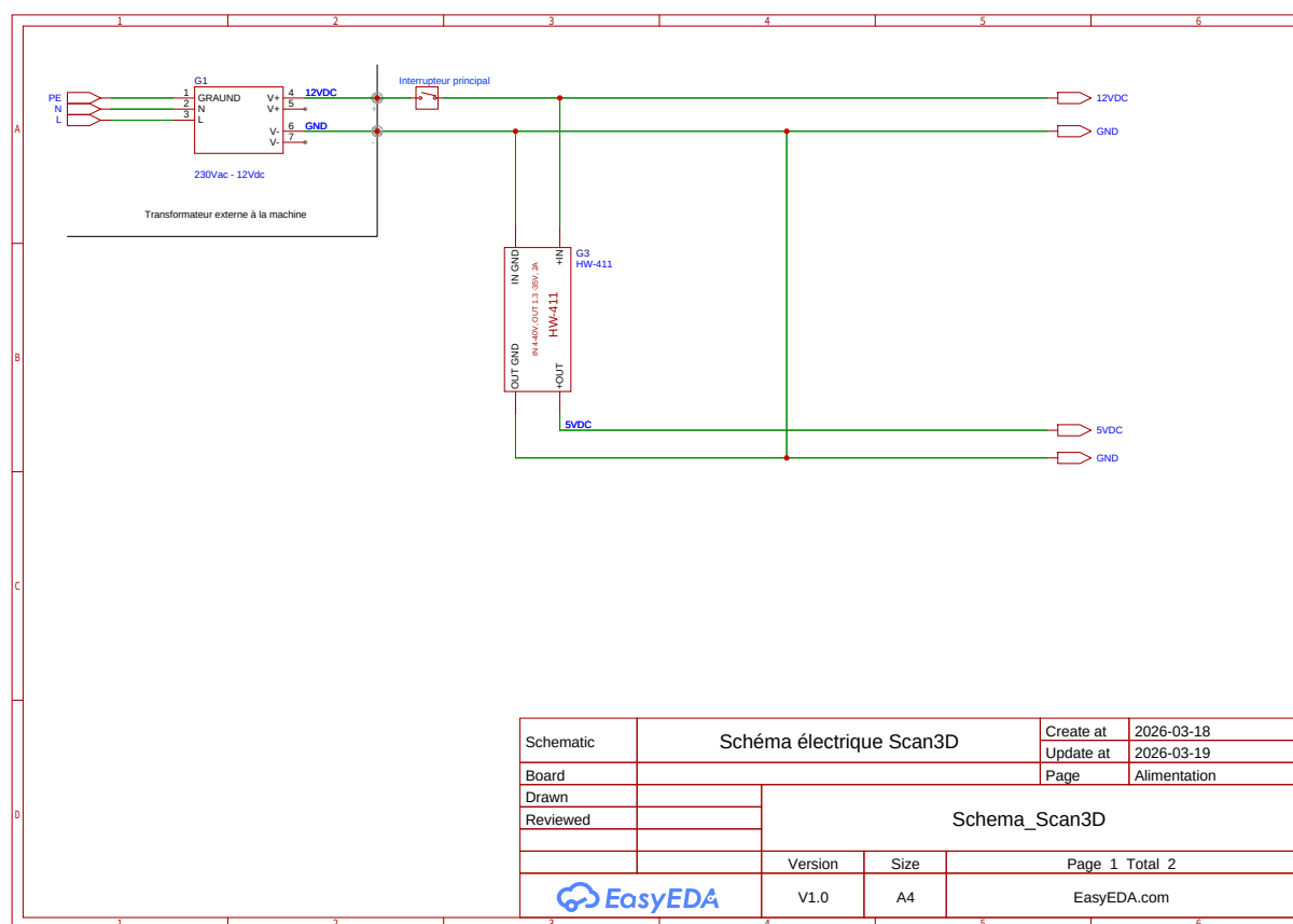
FIGURE 8 – Schéma électrique — étage d'alimentation.
