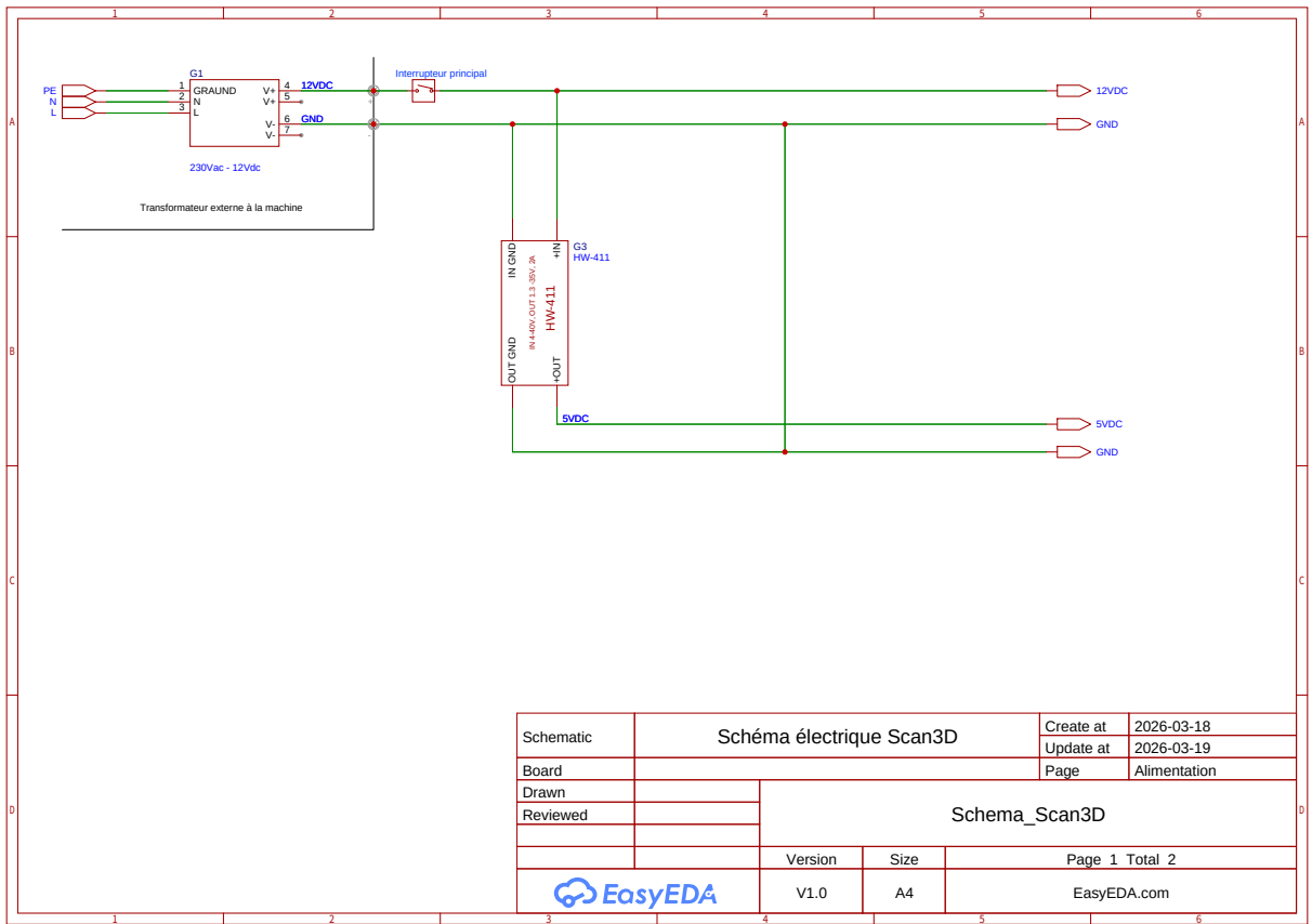
FIGURE 7 – Schéma électrique — étage d'alimentation.
