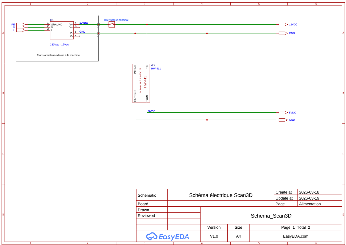
FIGURE 3 – Schéma électrique — étage alimétation électrique.
