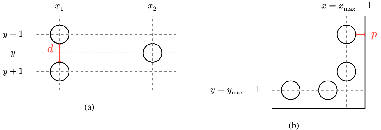
Abbildung 4: Veranschaulichung des Modells. Bezeichnungen in Rot stellen Werte in Millimetern dar.
