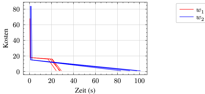
Abbildung 10: Ergebnisse Backtracking für Wandkonfigurationen w_1 und w_2 (min. Kosten jeweils 1)
