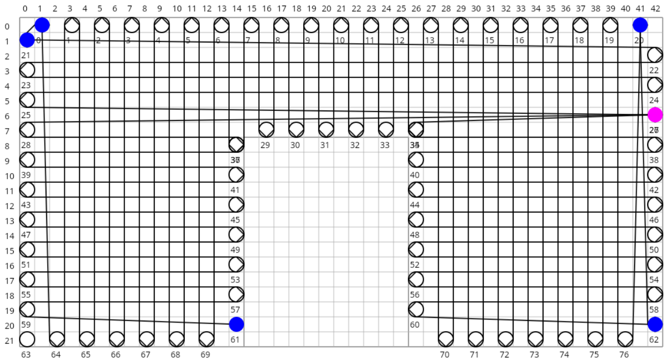
Abbildung 24: Annäherung p' an resultierende Garnstruktur am Beispiel von Wandkonfiguration w_4
