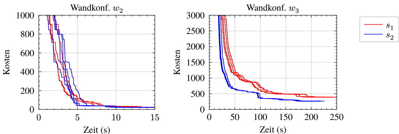
Abbildung 11: Ergebnisse für GA für Wandkonfiguration w_2 und w_3 mit Seeds s_1 und s_2
