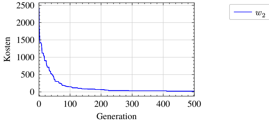
Abbildung 12: Ergebnisse GA für Wandkonfiguration w_2 (min. Kosten 21 nach 411 Generationen)
