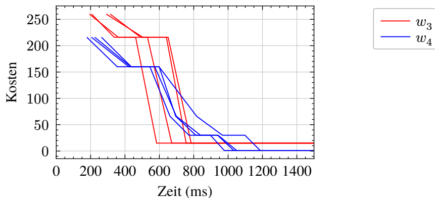
Abbildung 17: Ergebnisse teilroutenbasierter GA für Wandkonfigurationen w_3 und w_4 mit Seed s_1
