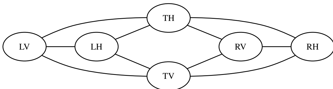
Abbildung 15: Teilrouten Graph
