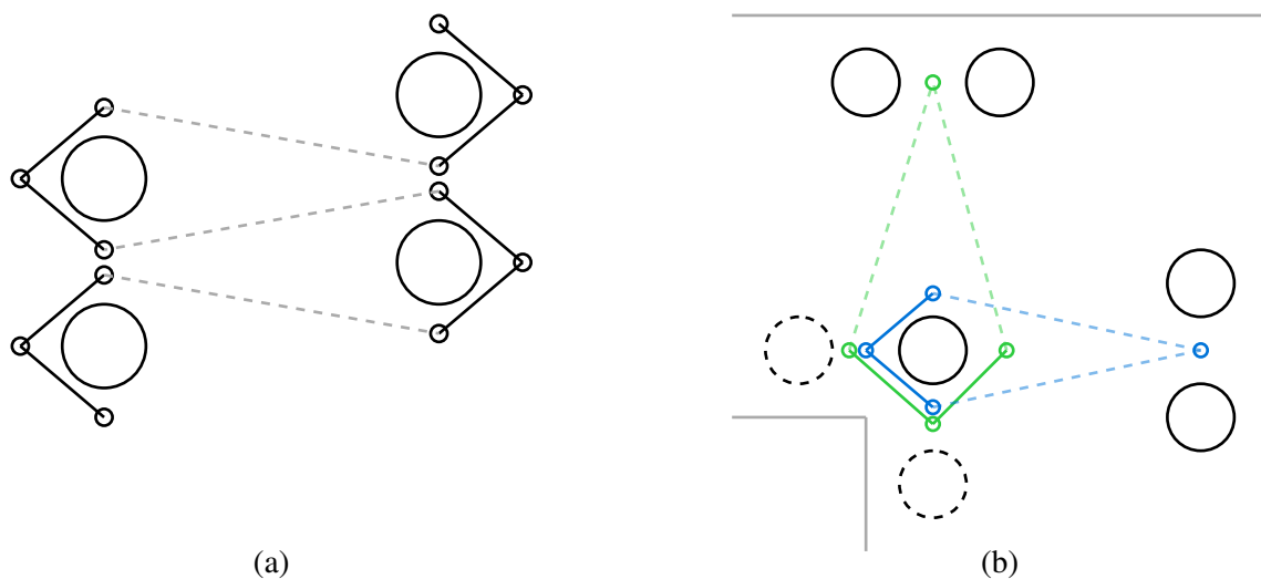
Abbildung 22: Positionen der Wegpunkte an den Umlenkelementen. Sowohl für Umlenkungen in Haupt- richtung (a) sowie an der oberen rechten Türecke (b).
