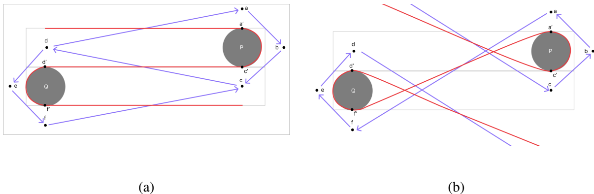
Abbildung 19: Pfad des Roboters (Blau) und daraus resultierende Garnstruktur (Rot) um zwei Umlenkelemente mit korrekter Umlaufrichtung (links) und vertauschter Umlaufrichtung (rechts)
