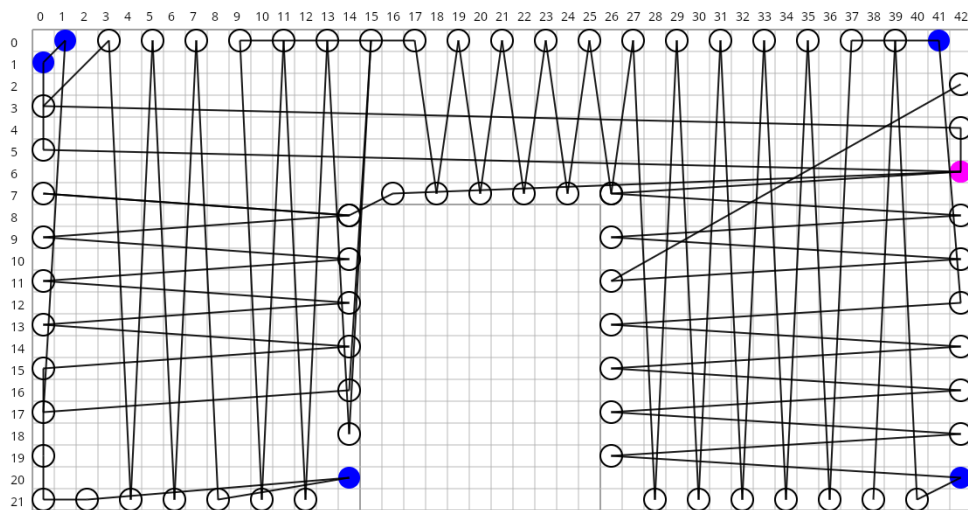
Abbildung 13: Von GA berechnete Route für Wand w_4 unter Seed s_2
