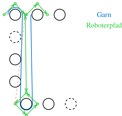
Abbildung 23: Vollständige Umlenkung zur Vermeidung einer Kollision mit einem Umlenkelement. In Grün dargestellt der Roboterpfad und in Blau die resultierende Garnstruktur
