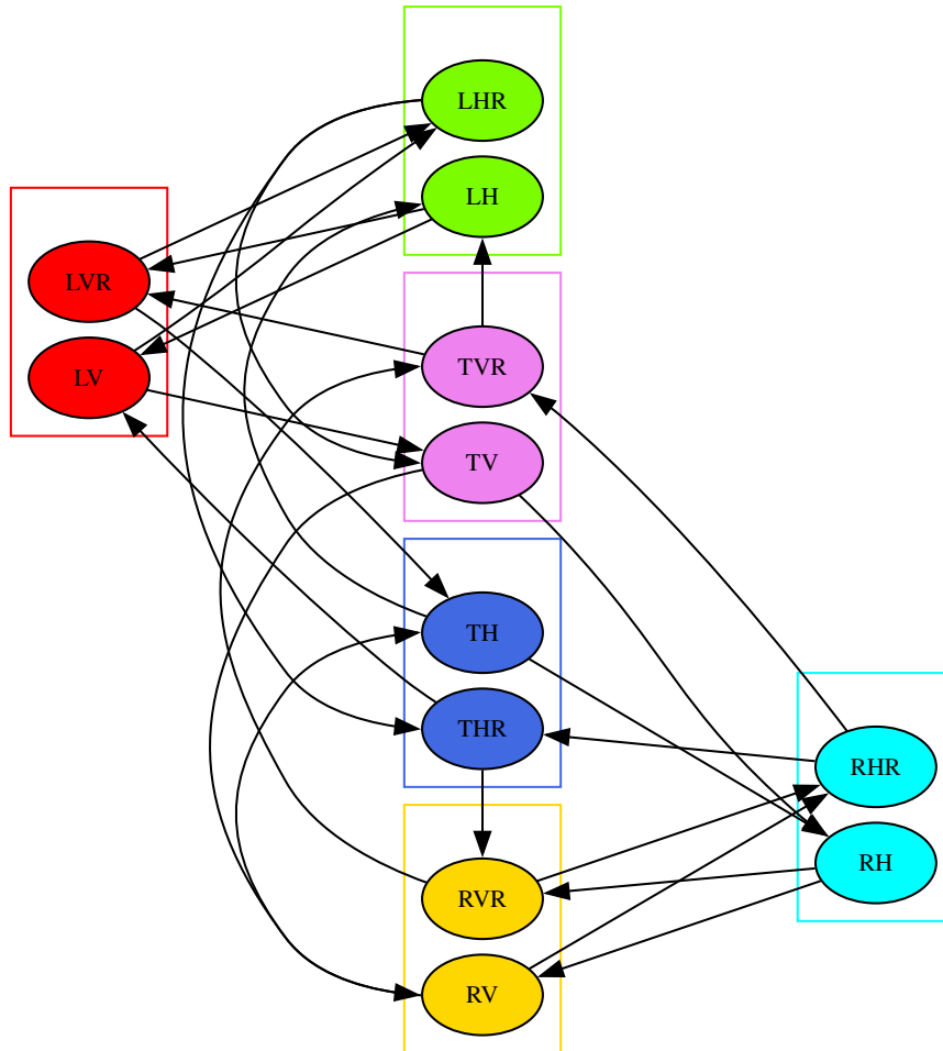
Abbildung 16: Teilrouten Graph
