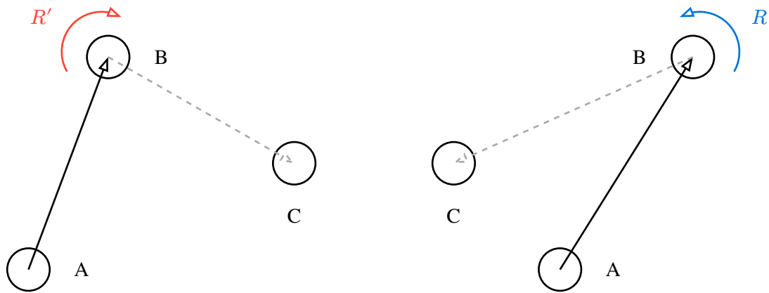
Abbildung 20: Vektorbasierte Bestimmung der Umlaufrichtung um einen Knoten B basierend auf seinem Vorgänger und Nachfolger
