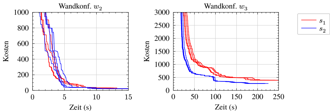
Abbildung 12: Ergebnisse für GA für Wandkonfiguration w_2 und w_3 mit Seeds s_1 und s_2
