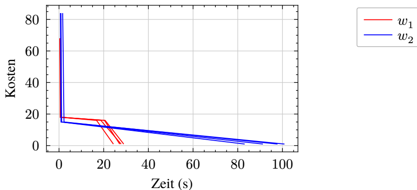
Abbildung 11: Ergebnisse Backtracking für Wandkonfigurationen w_1 und w_2 (min. Kosten jeweils 1)
