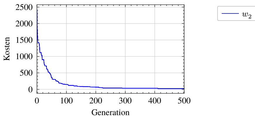
Abbildung 13: Ergebnisse GA für Wandkonfiguration w_2 (min. Kosten 21 nach 411 Generationen)
