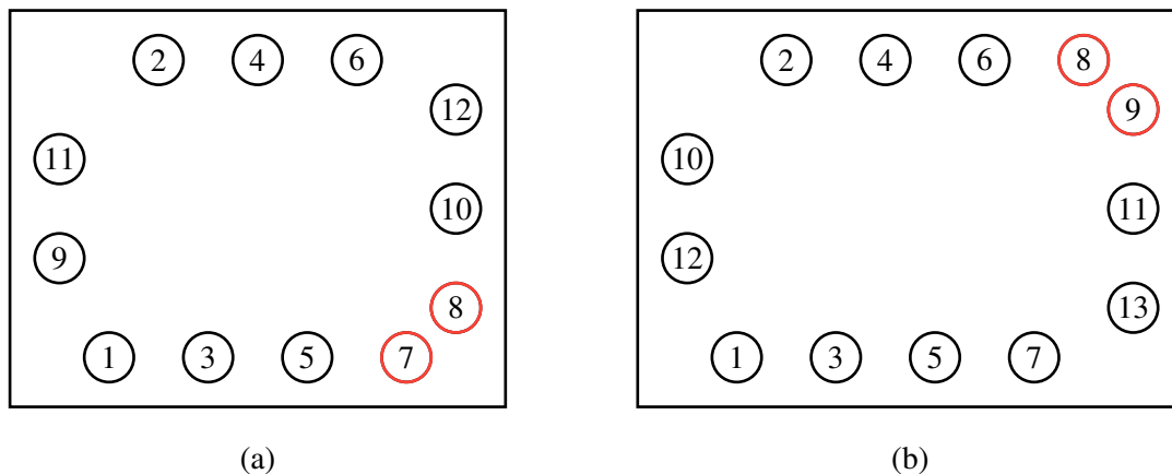
Abbildung 5: Reihenfolge der Positionierung der UE im aktuellen Ansatz des CBT für einfache Wände ohne Tür- oder Fensterausschnitt. In Rot sind die UE der Sonderstelle markiert.
