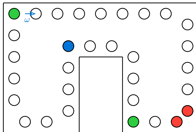
Abbildung 8: Kleine Wandkonfiguration mit korrekt platzierten Umlenkelementen. In Rot dargestellt eine Sonderstelle, in Grün optionale UE und in Blau das UE, welches den oberen Versatz \omega bestimmt.
