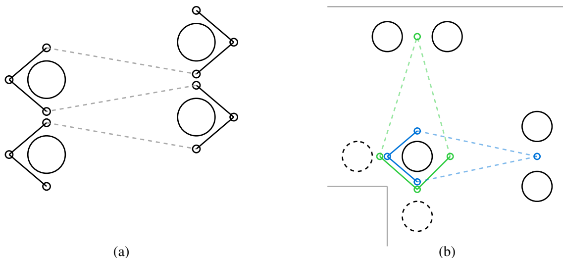
Abbildung 23: Positionen der Wegpunkte an den Umlenkelementen. Sowohl für Umlenkungen in Hauptrichtung (a) sowie an der oberen rechten Türecke (b).
