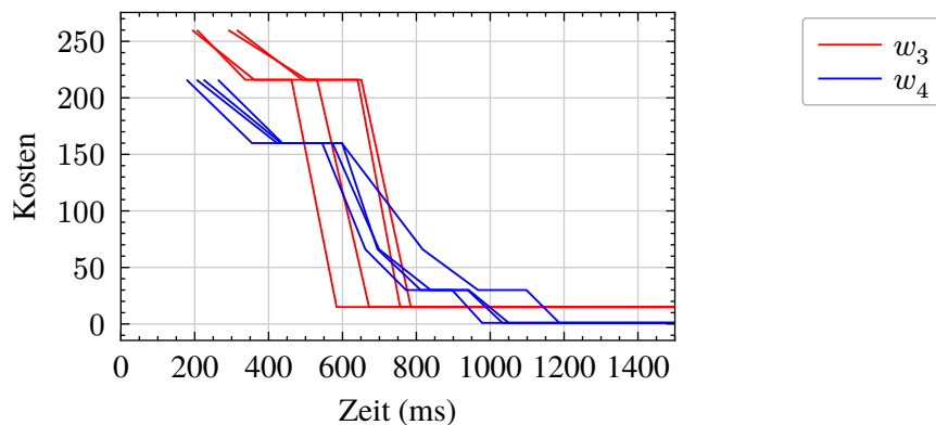
Abbildung 18: Ergebnisse teilroutenbasierter GA für Wandkonfigurationen w_3 und w_4 mit Seed s_1
