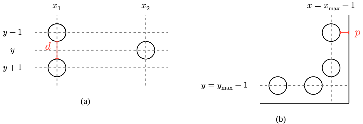
Abbildung 4: Veranschaulichung des Modells. Bezeichnungen in Rot stellen Werte in Millimetern dar.
