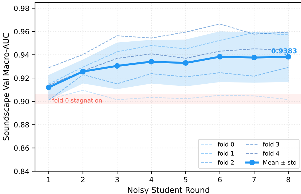
EfficientNet-B0
