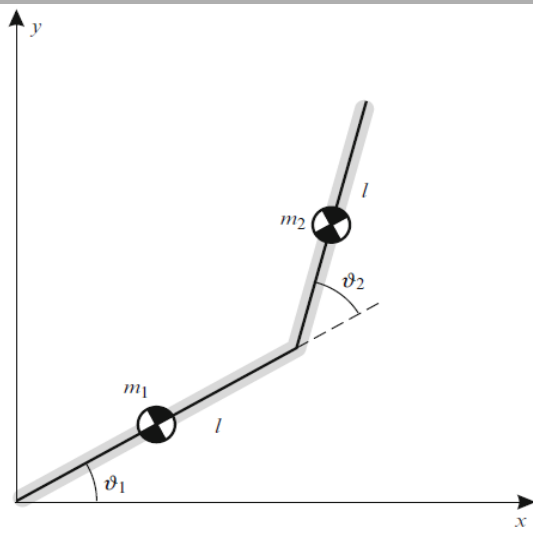
Fig 5.12. Robot Planar 2 GDL
