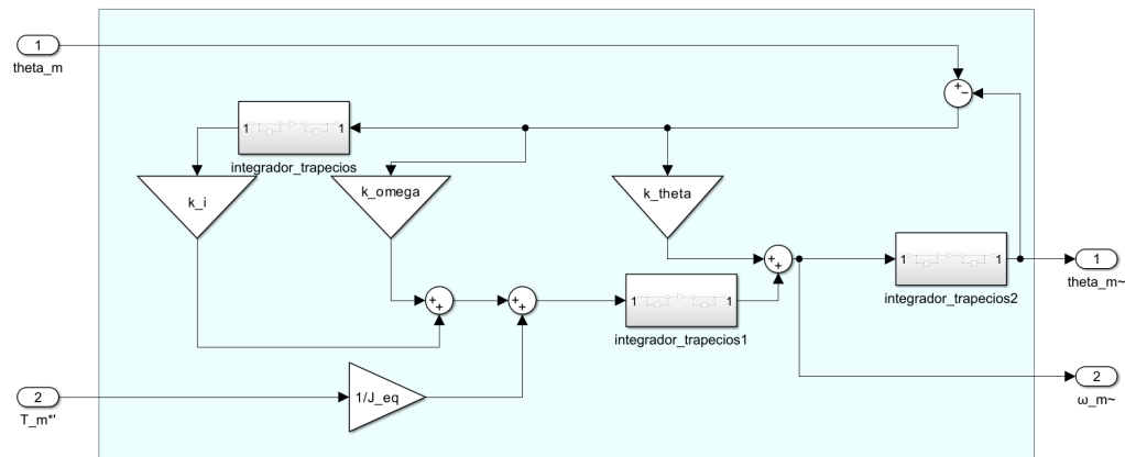
Figura 86: bloques observador reducido discreto
