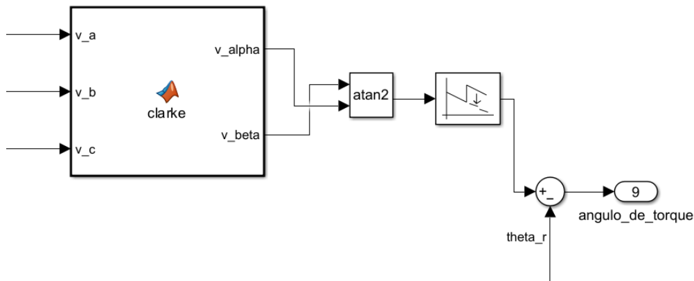
Figura 28: bloques correspondientes al cálculo de \delta(t)
