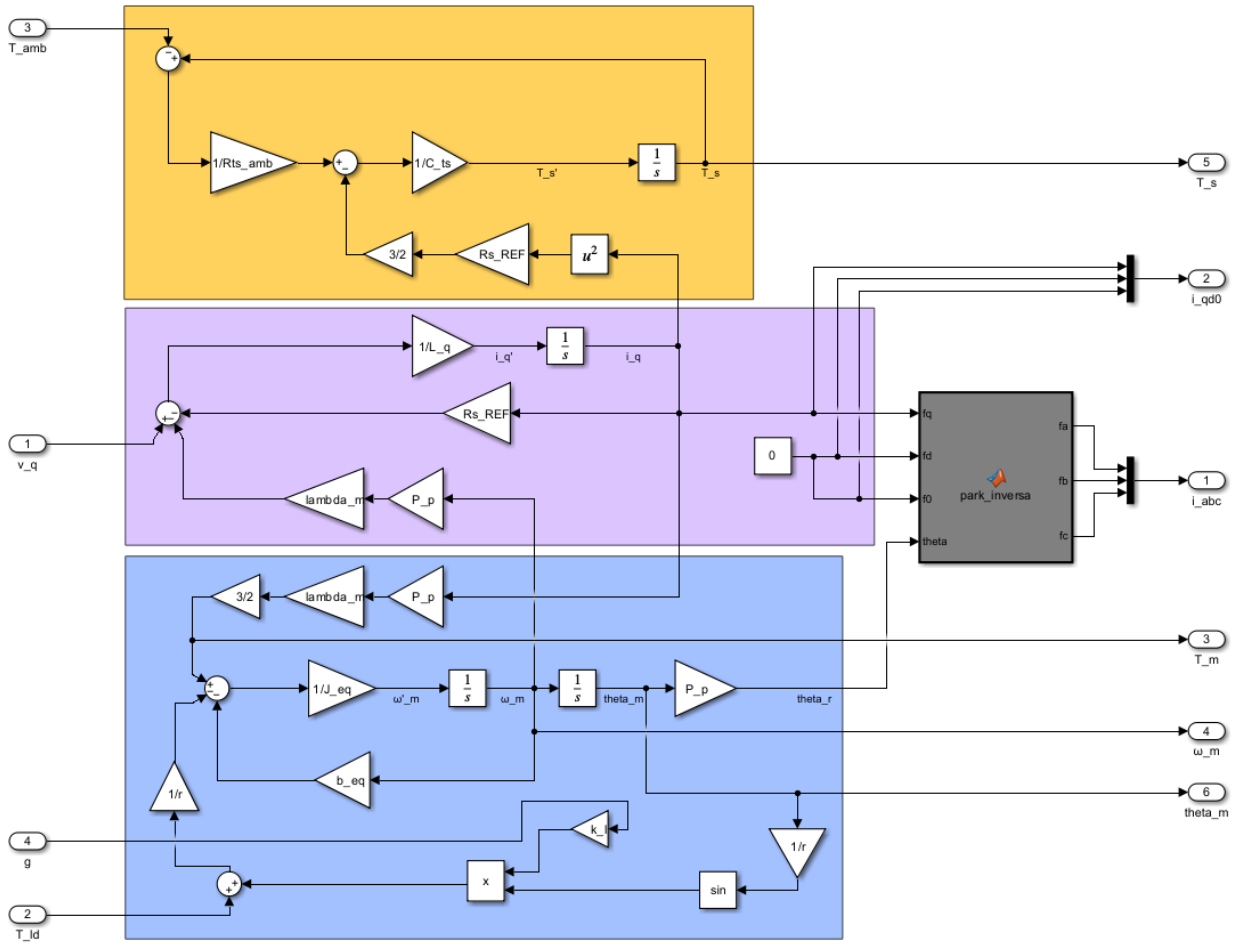
Figura 8: sistema LTI equivalente por retroalimentación NL
