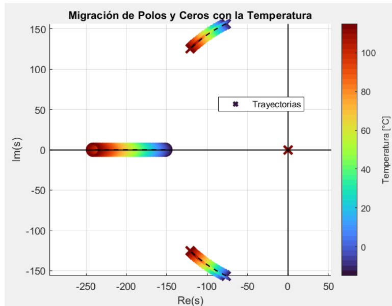
Figura 13: migración de polos y ceros variando la temperatura estatórica
