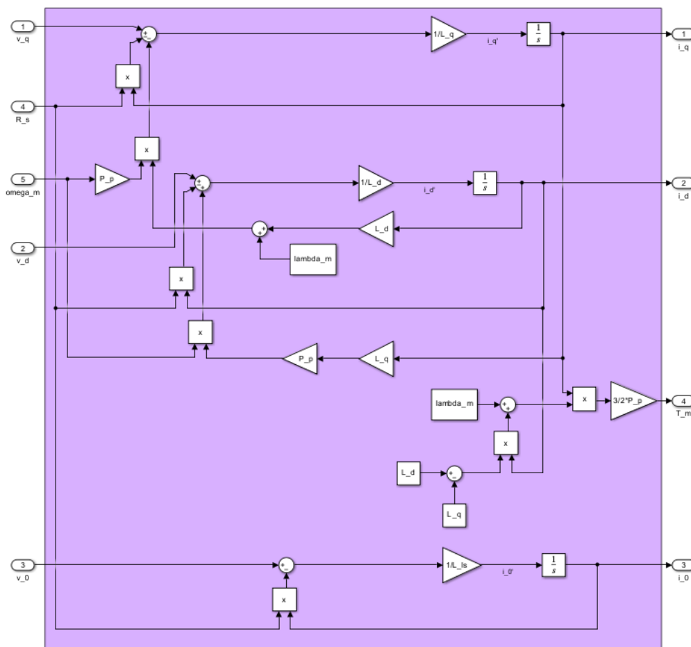
Figura 4: Subsistema electromagnético
