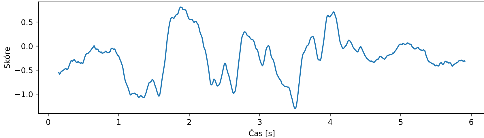
Priebeh skóre
