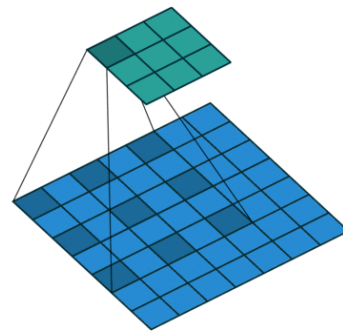
\delta = 2
