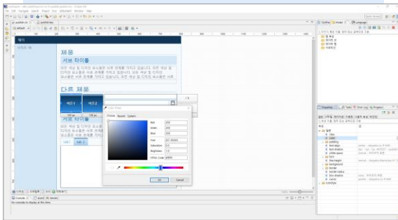
eXBuilder6 개발환경 내 디자인 편집기
