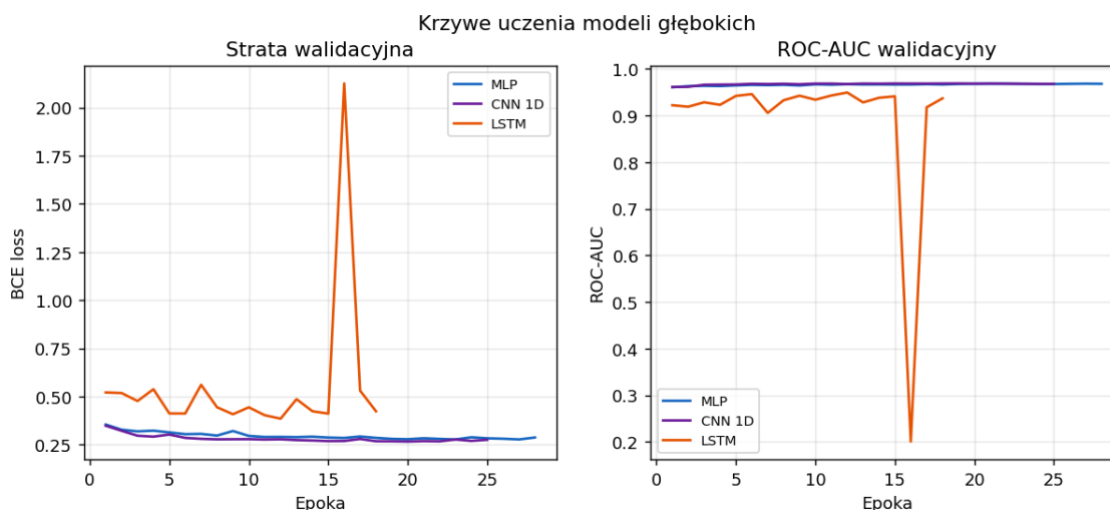
Rysunek 7. Krzywe uczenia modeli głębokich (strata i ROC-AUC walidacyjny).
