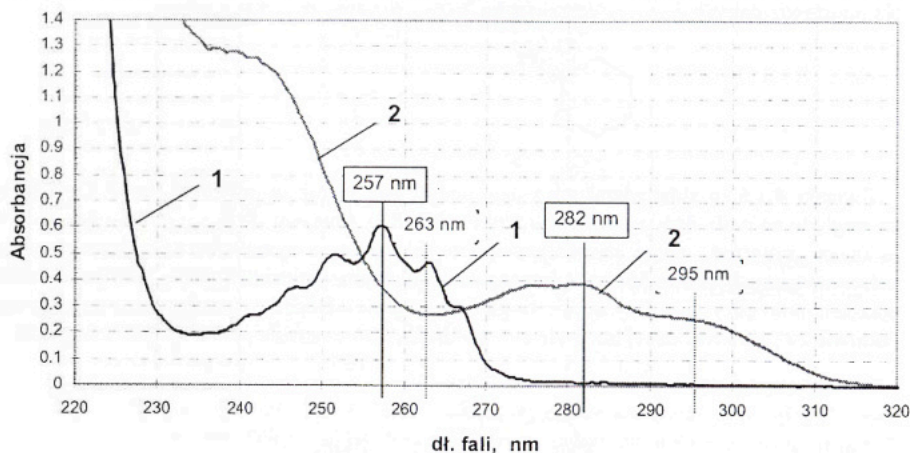
Rys. 2. Wyznaczanie analitycznych długości fali
