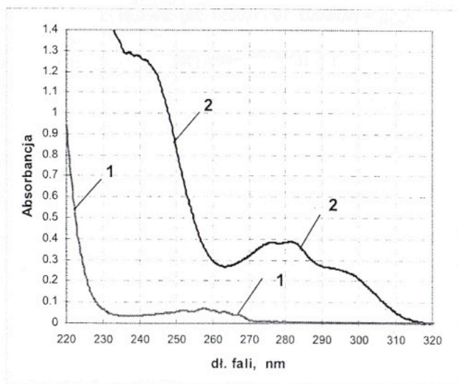
Rys. 3. Widma absorpcji fenyloalaniny i tyrozyny (stężenie substancji 50 \mu\text{g mL}^{-1} , kuweta 1 cm)
