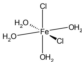
Izomer cis
