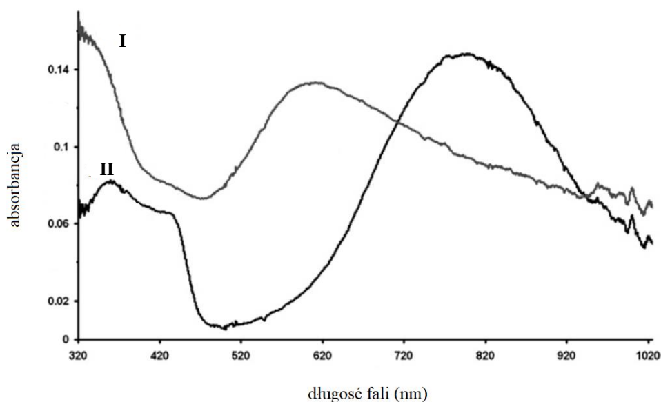
Rys. 1 Widma UV-Vis formy I i II polianiliny.
