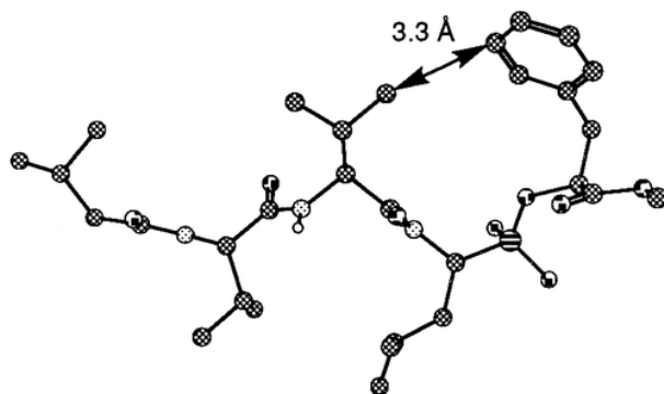
Rys. 1. Model przestrzenny inhibitora penicilopepsyny w konformacji aktywnej.
