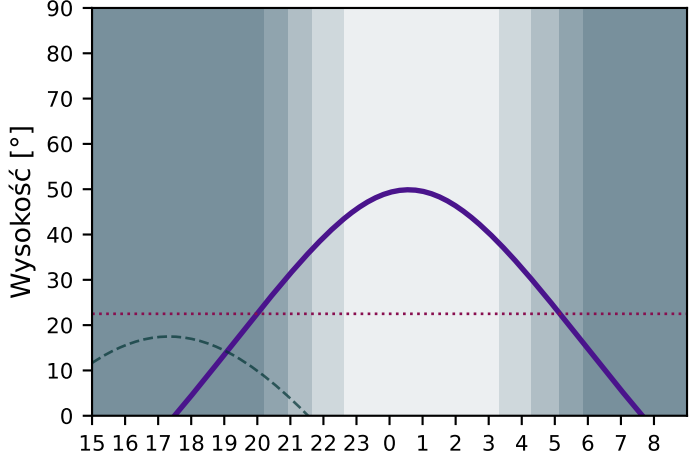
Wysokość obiektu 18.08. Max: 09.09/7.5h
