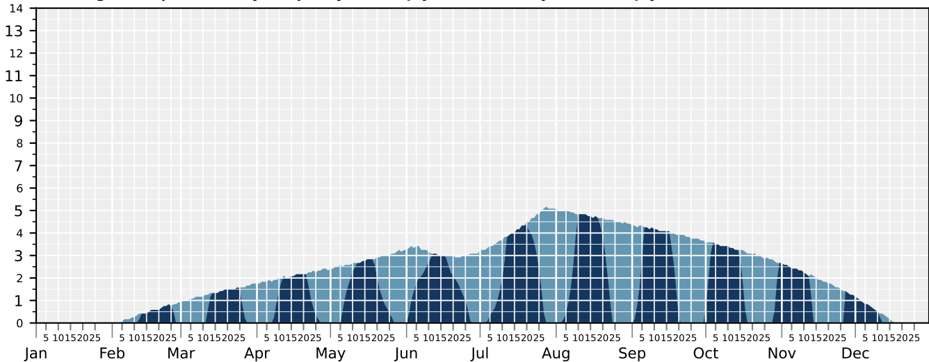
Suma godzin jakościowych (jasny: z Księżycem, ciemny: bez Księżycyca)
