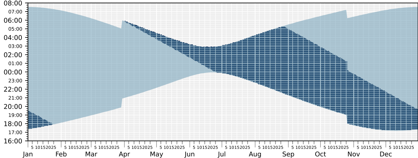
Suma godzin jakościowych (jasny: z Księżycem, ciemny: bez Księżyca)
