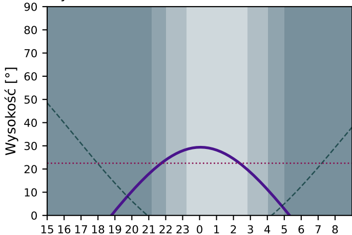
Wysokość obiektu 13.07. Max: 13.07/3.5h
