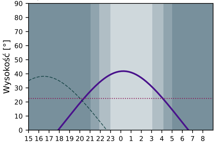
Wysokość obiektu 18.07. Max: 10.08/4.8h
