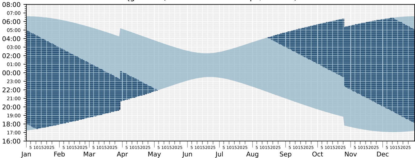
Suma godzin jakościowych (jasny: z Księżycem, ciemny: bez Księżyca)
