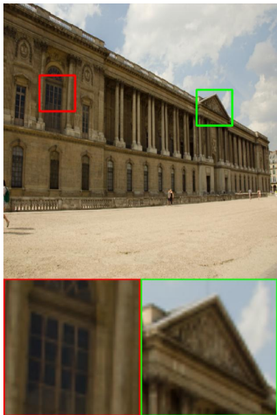
Zero-DCE
