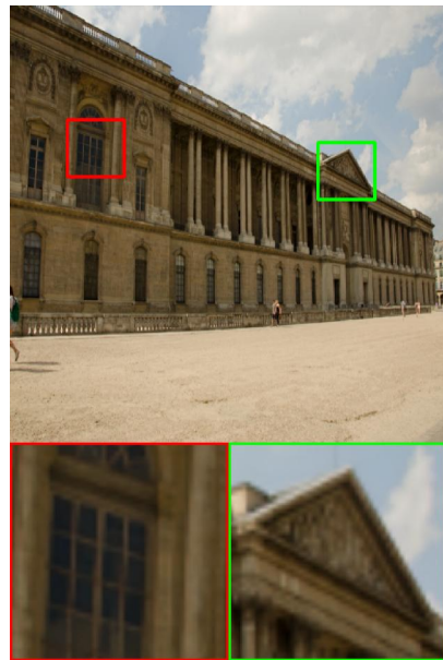
LLFlow
