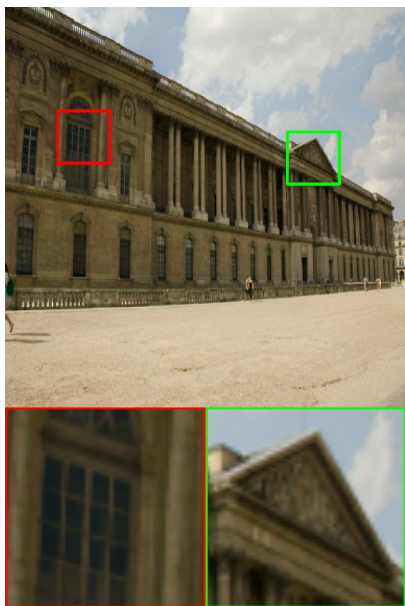
LIME
