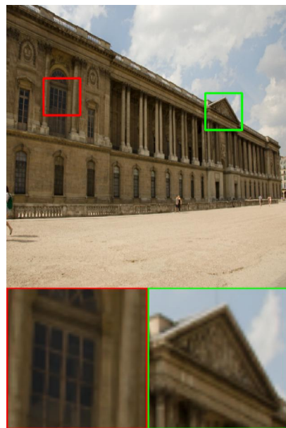
LLFlow
