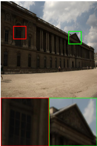
Input
