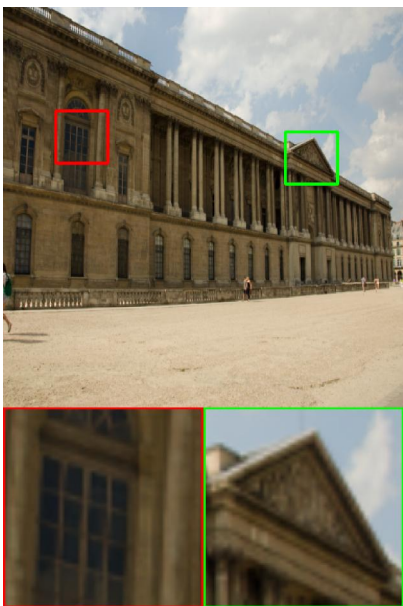
Input
