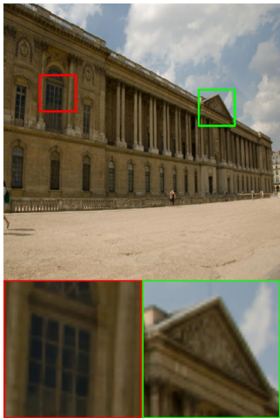
LIME
