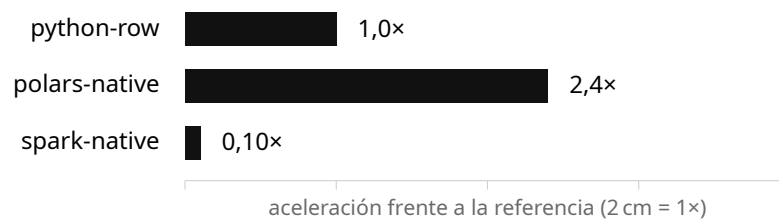
Figura 4 Aceleración frente a la referencia en el perfil small : Polars ~2,4x con el mismo resultado; Spark local queda en 0,10x en esta escala por su coste de arranque. Tiempos absolutos en la tabla anterior.
