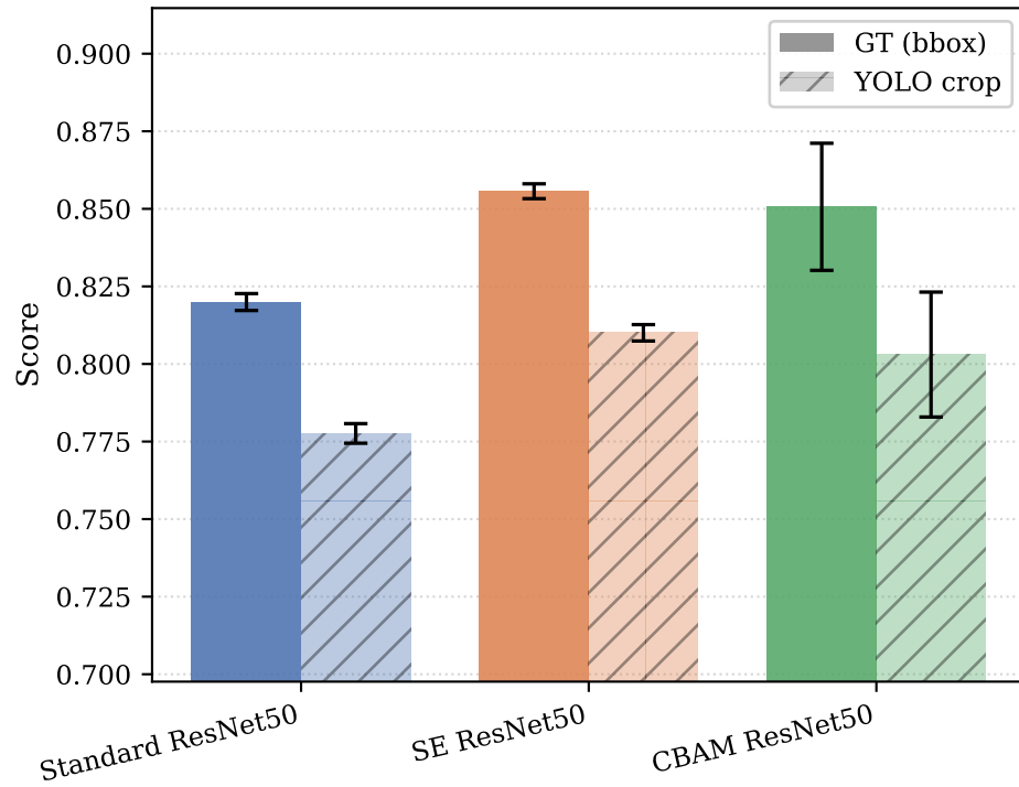
Macro F1
