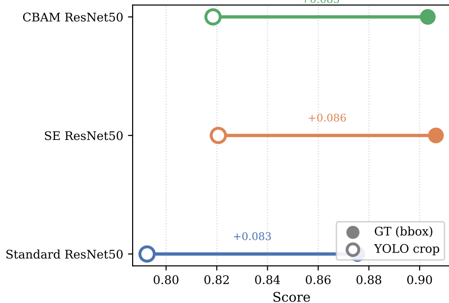
Macro F1
