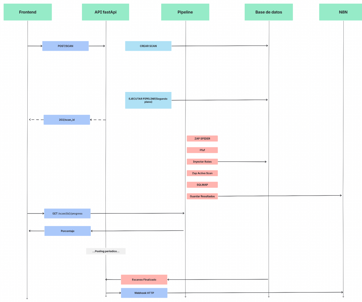
Figura 4 (ampliada). Diagrama de secuencia UML. Elaboración propia.
