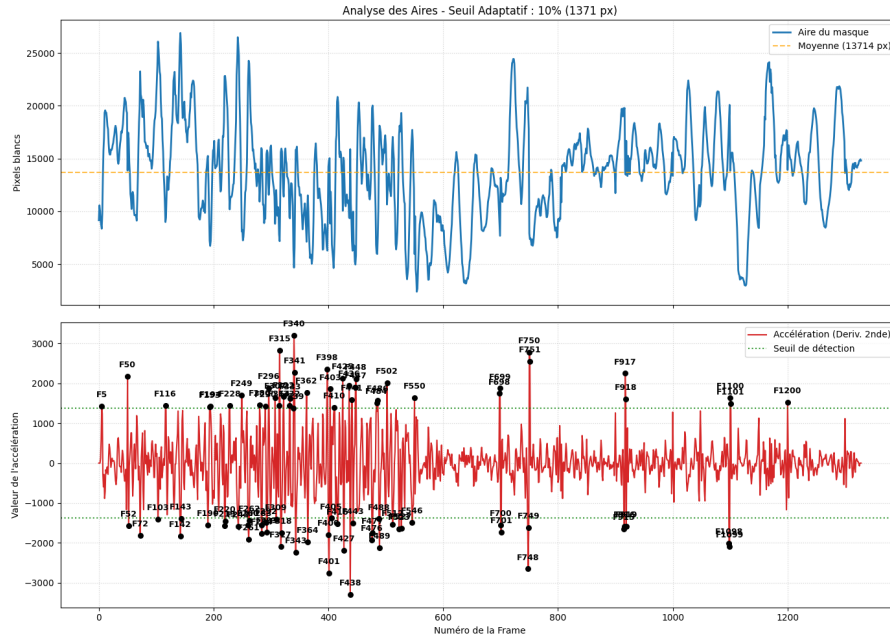
Figure 9 – Évolution temporelle des aires des masques et dérivée seconde associée.
