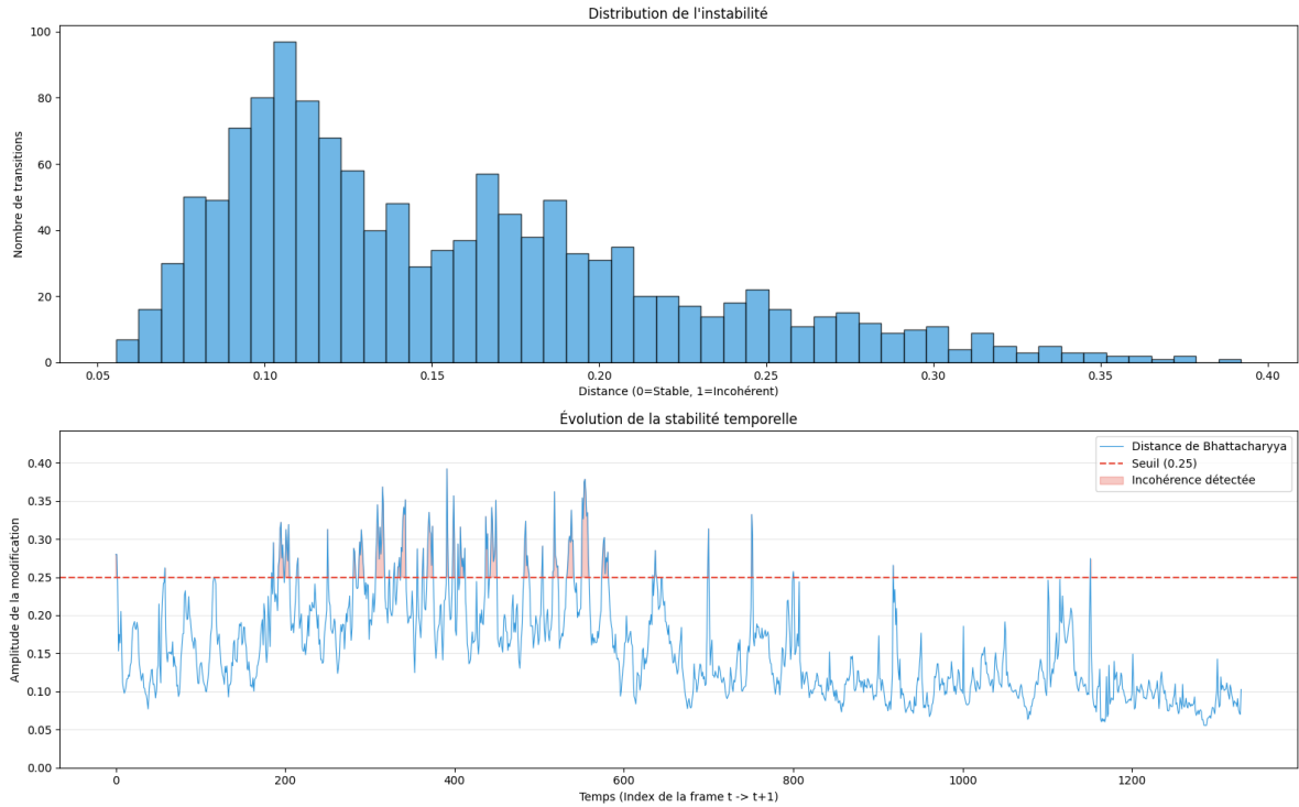
Figure 12 – Distribution et évolution temporelle de la distance de Bhattacharyya avec overlay de masques voisins.
