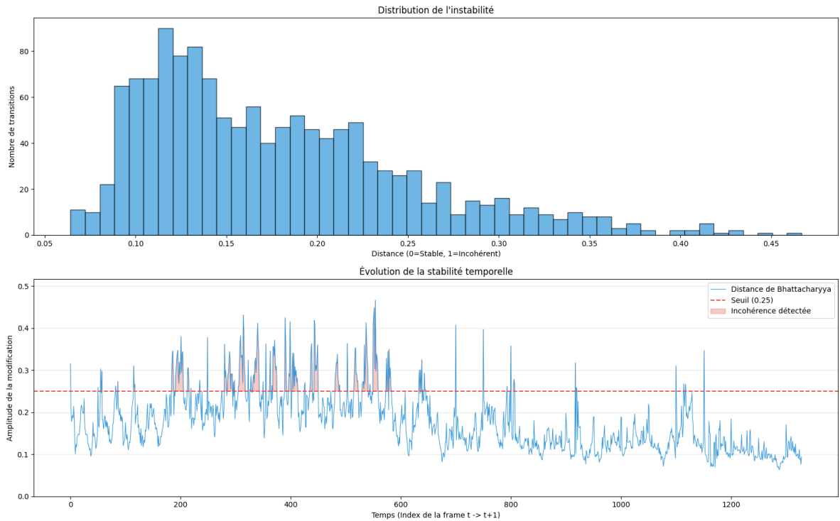
Figure 11 – Distribution et évolution temporelle de la distance de Bhattacharyya sans overlay.
