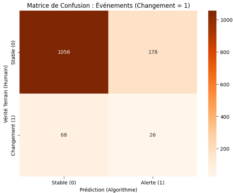
Figure 14 – Matrice de confusion associée à la détection des changements d’état, sans overlay.
