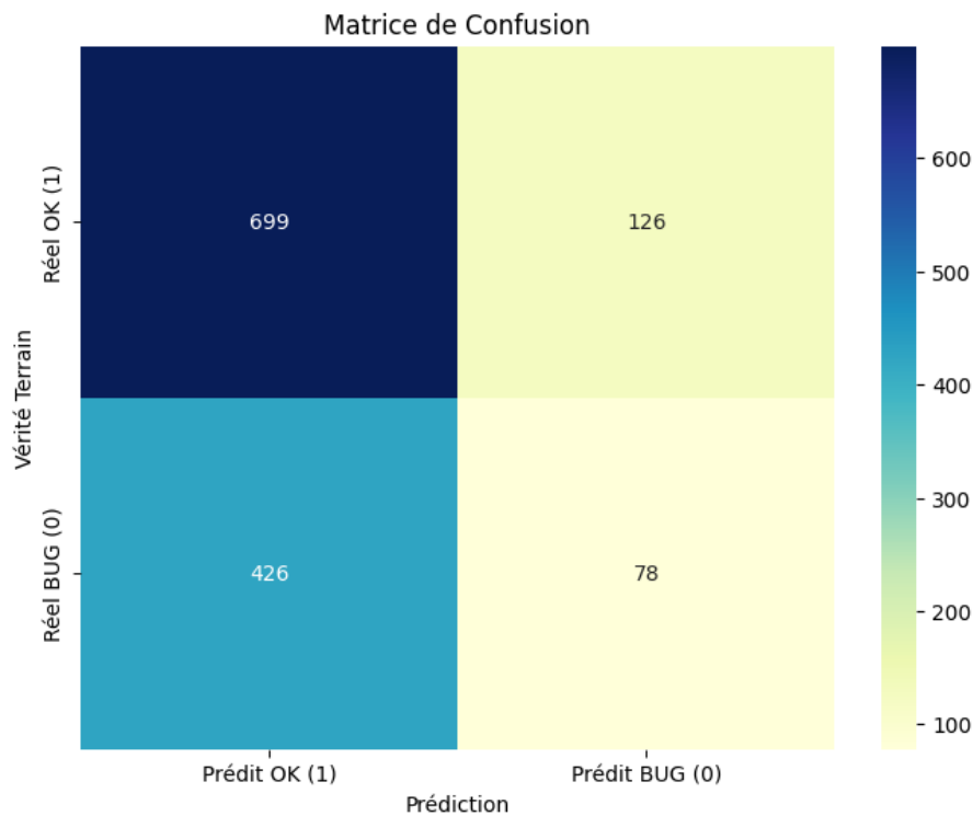
Figure 13 – Matrice de confusion associée à la détection des frames correctes et incorrectes, sans overlay.
