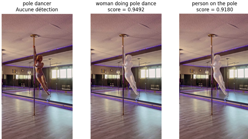
Figure 8 – Exemple de calibration d’un prompt texte dans la V4 basée sur SAM 3.
