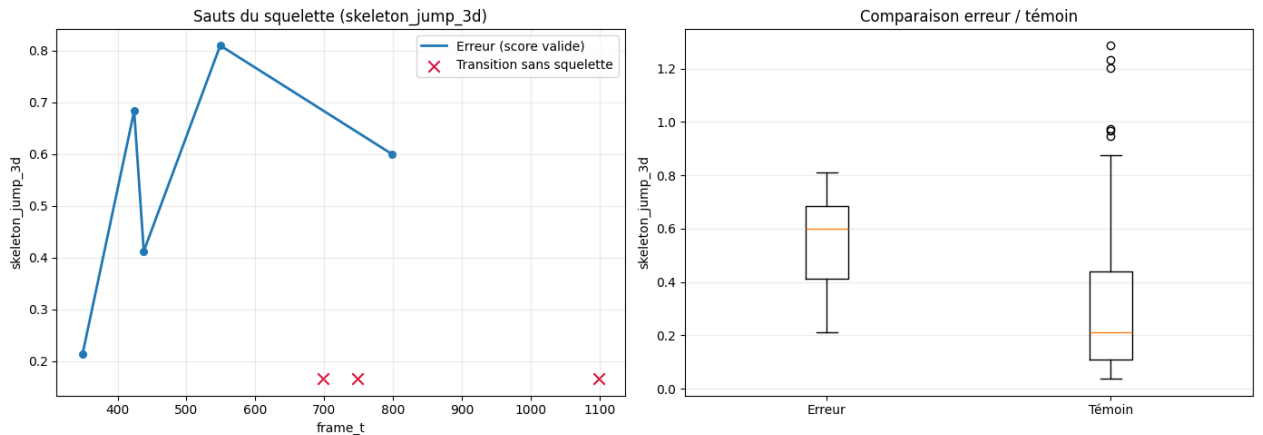
Figure 15 – Évolution des sauts du squelette estimés par SAM 3D Body sur les transitions anormales détectées (gauche) et comparaison entre transitions d’erreur et transitions témoins (droite). Les croix rouges correspondent aux transitions pour lesquelles aucun squelette valide n’a pu être reconstruit.
