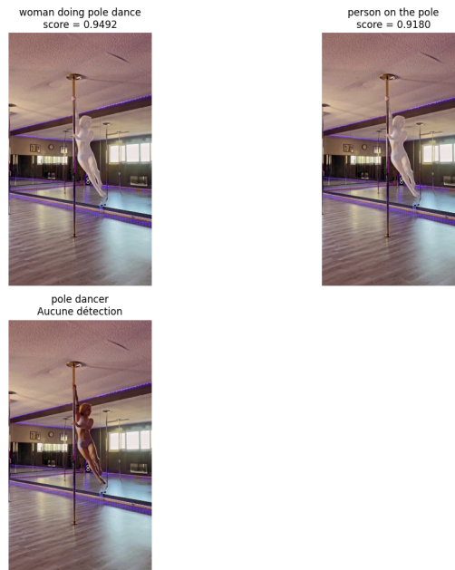
Figure 17 – Exemple de calibration d'un prompt texte dans la version exploratoire V4 basée sur SAM 3 .
