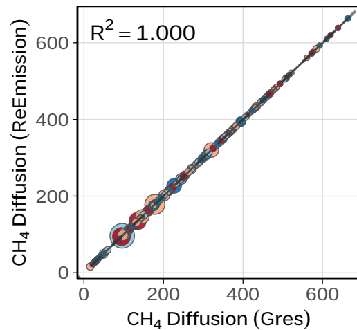
CH 4 Diffusion
