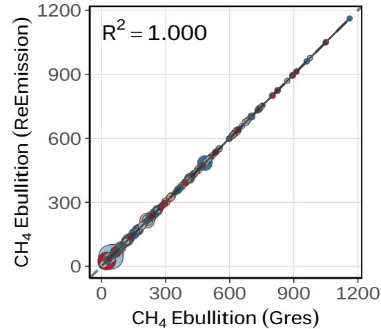
CH 4 Ebullition
