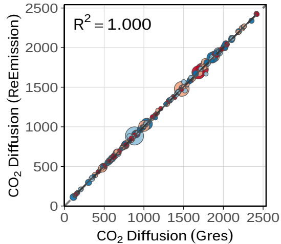
CO 2 Diffusion
