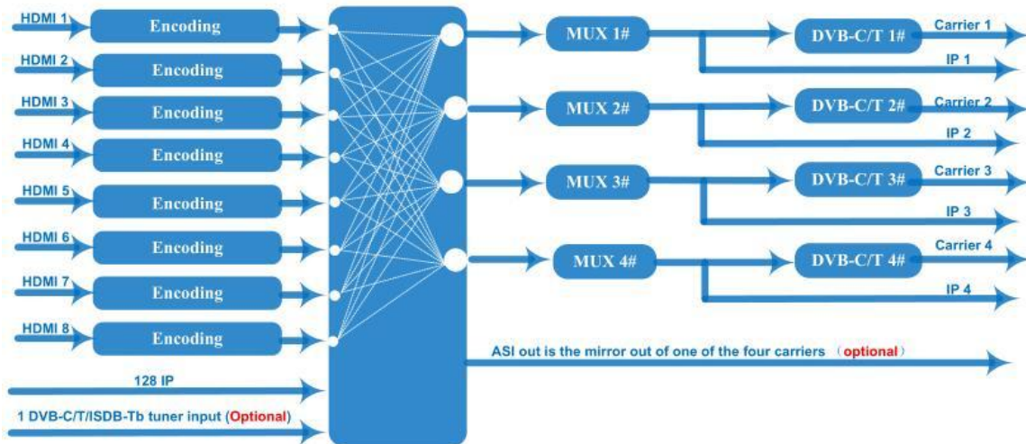
NDS3524S
