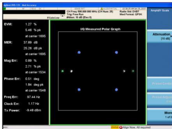
Figure 4 MER (QPSK)
