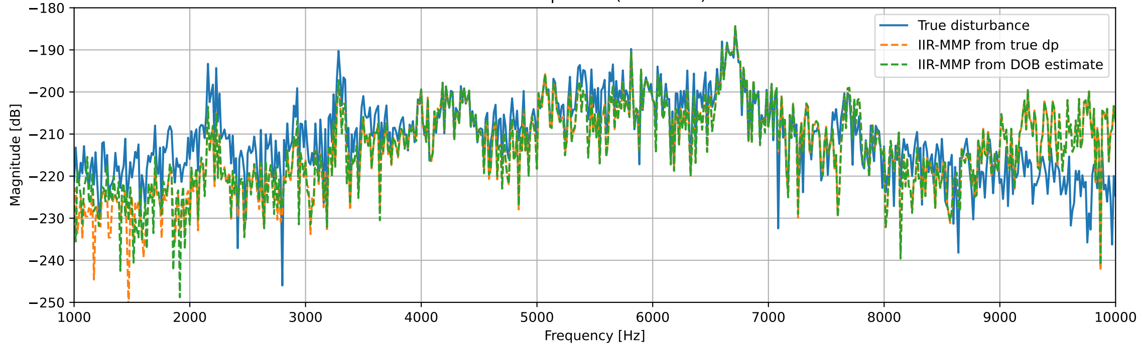
FFT comparison ( t > 0.01 s)
