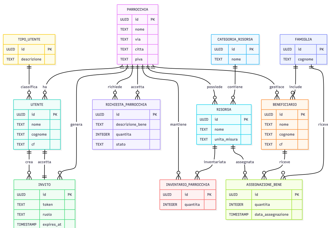
Figura 1: Schema ER Database KARIS
