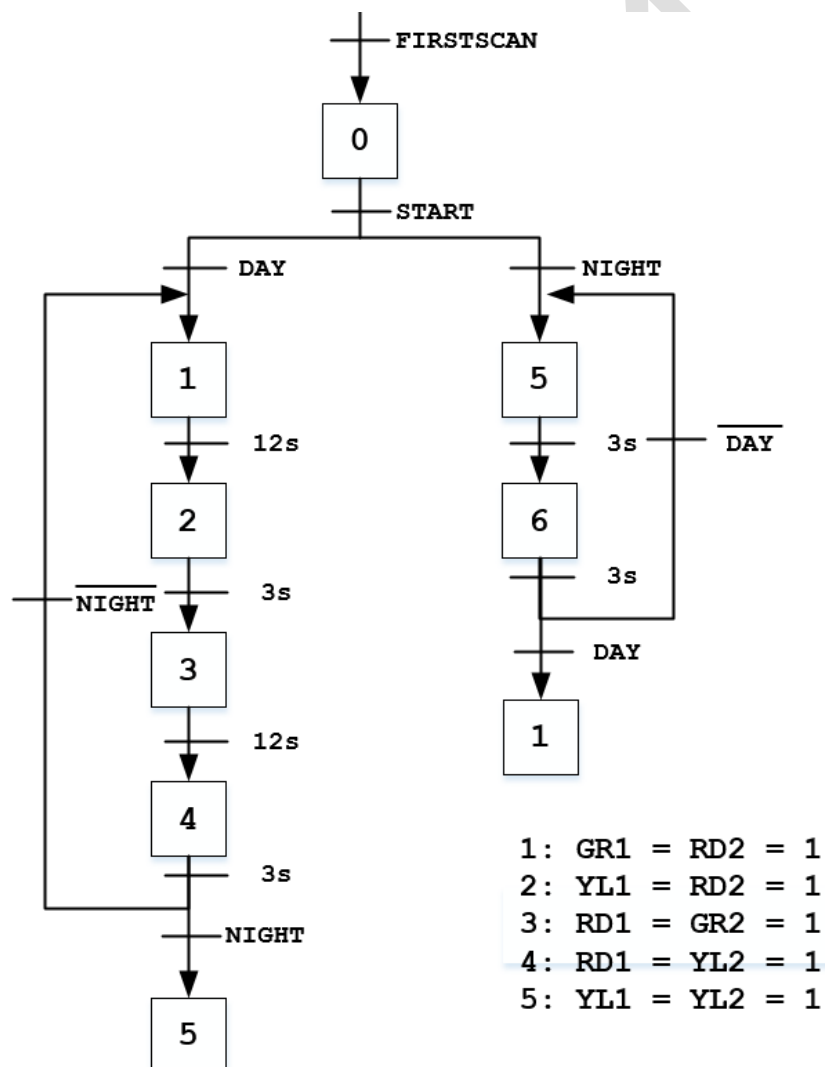
Figure 2.1. The Grafcet
