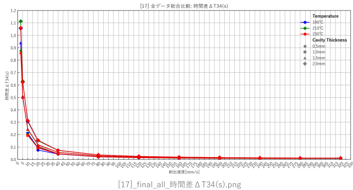
バージンPP（pp）・最大値版・Alldata
