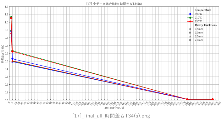
粉砕材混合PP（mixpp）・最大値版・3data
