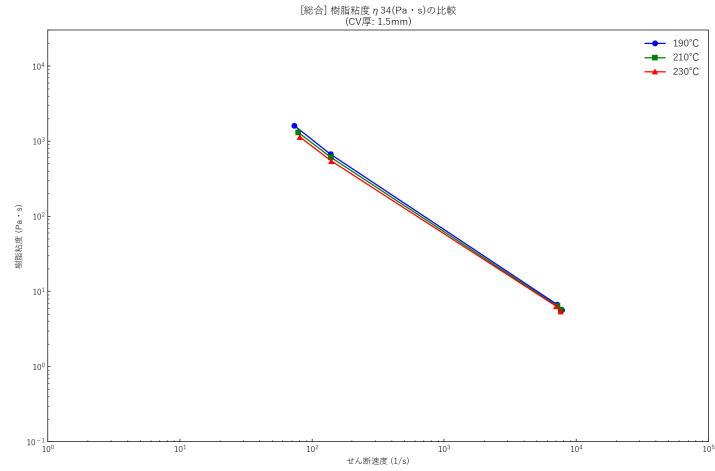
バージンPP（pp）・最大値版・3data
