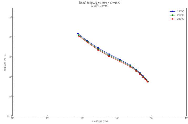
バージンPP（pp）・最大値版・Alldata
