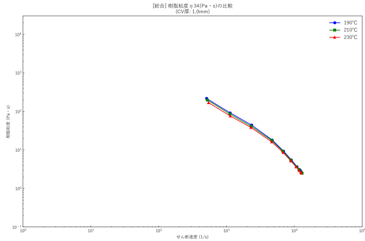
粉碎材混合PP（mixpp）・最大値版・Alldata
