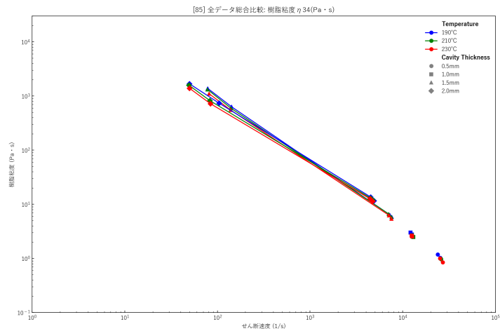
粉碎材混合PP（mixpp）・最大値版・3data
