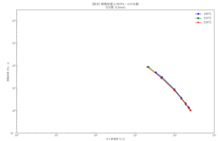
粉碎材混合PP（mixpp）・最大値版・5data
