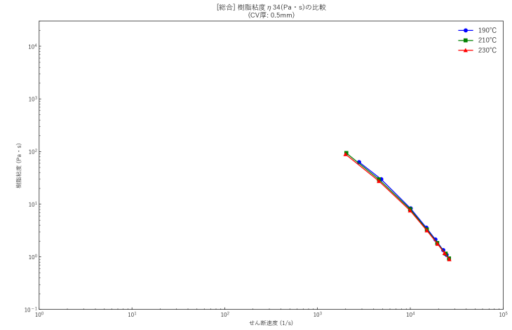
バージンPP（pp）・最大値版・5data
