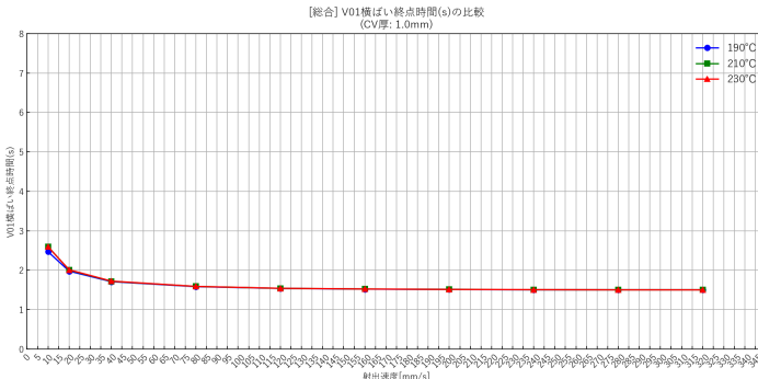
粉砕材混合PP (mixpp) ・ V01横ばい終点版 ・ Alldata
