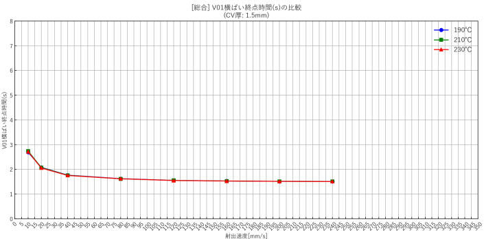
粉砕材混合PP（mixpp）・V01横ばい終点版・5data
