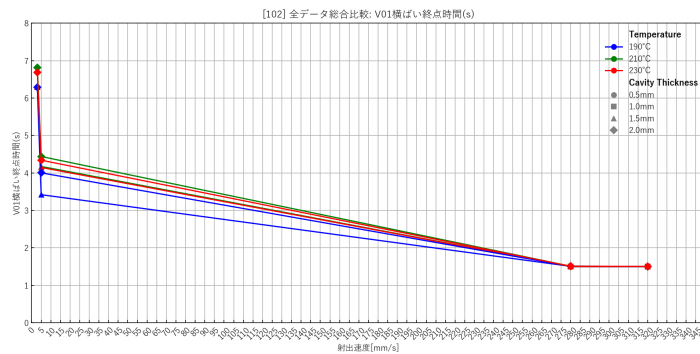
粉砕材混合PP（mixpp）・V01横ばい終点版・3data
