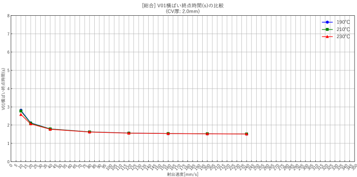
バージンPP（pp）・V01横ばい終点版・5data
