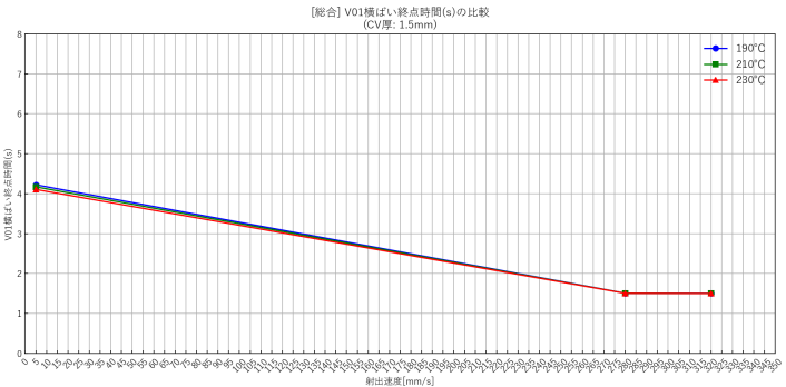
バージンPP（pp）・V01横ばい終点版・3data
