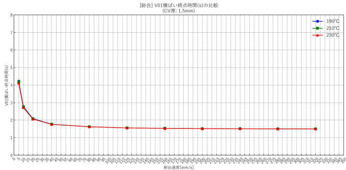
バージンPP（pp）・V01横ばい終点版・Alldata
