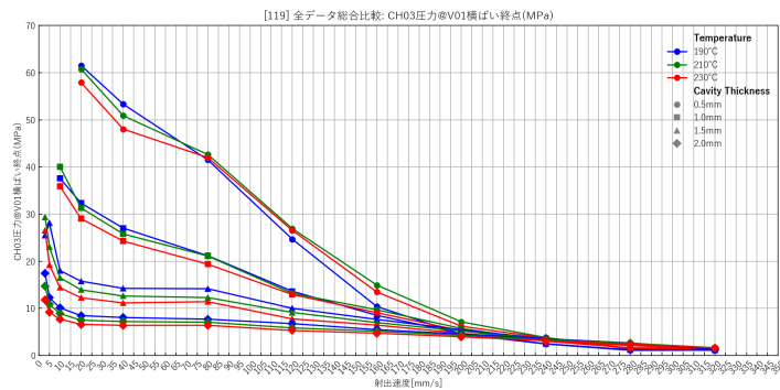
粉碎材混合PP（mixpp）・V01横ばい終点版・Alldata
