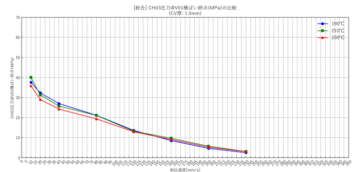
粉碎材混合PP（mixpp）・V01横ばい終点版・5data
