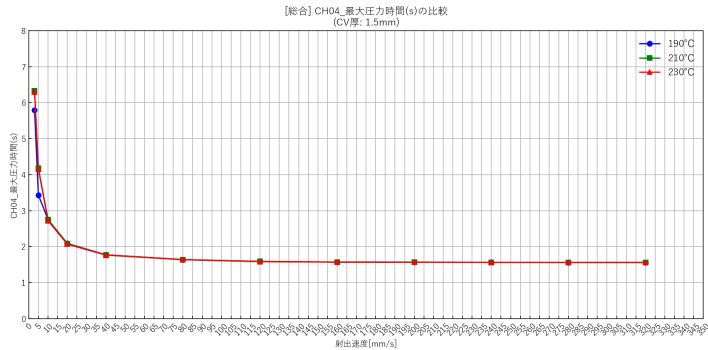
[148]_CV1.5_sum_CH04_最大圧力時間(s).png
