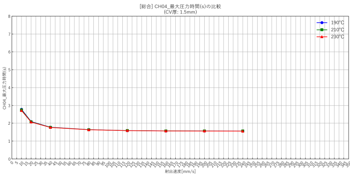
[148]_CV1.5_sum_CH04_最大圧力時間(s).png
