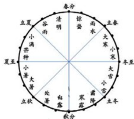
图2 二十四节气
