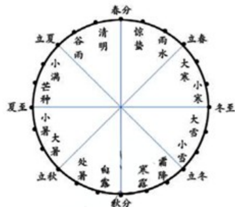
图2 二十四节气
