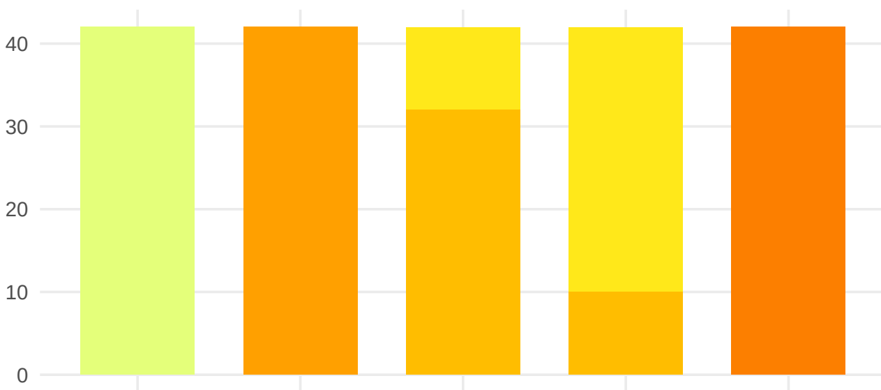
Deserialize
