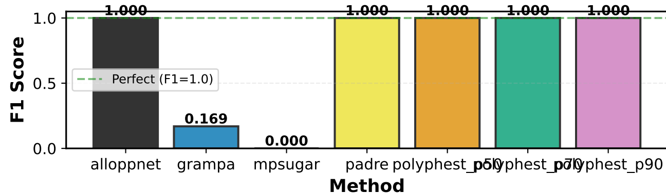
Polyploid Identification F1 Score
