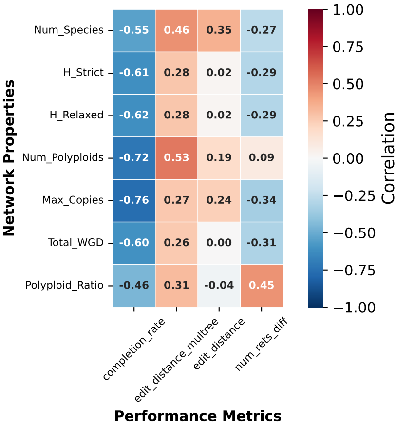
polyphest_p90
