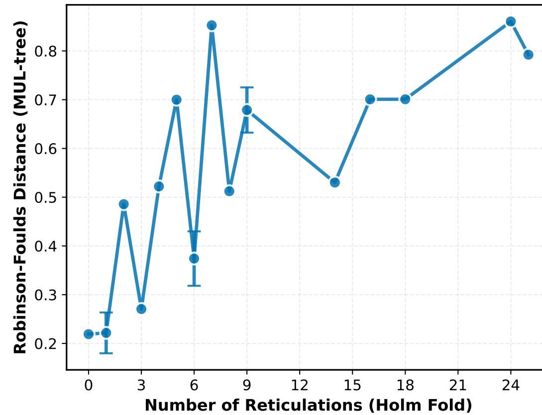
polyphest_p70
