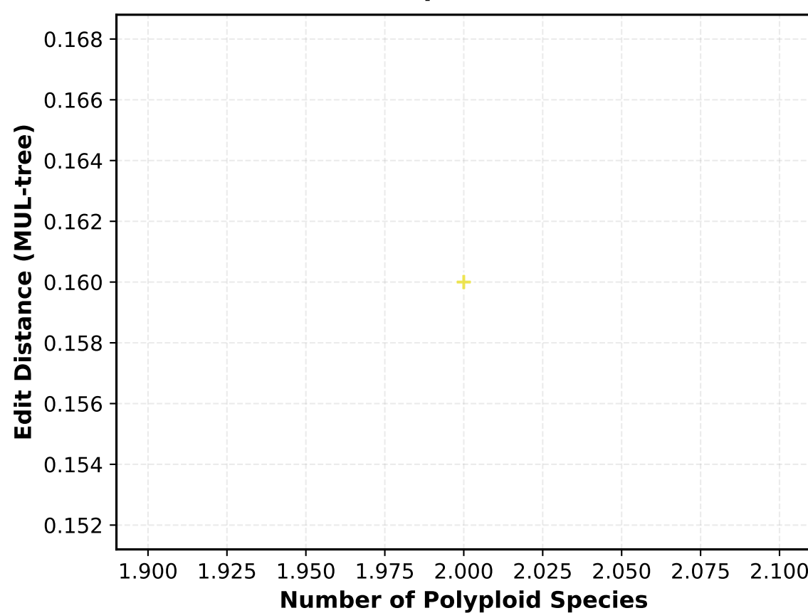
polyphest_p90
