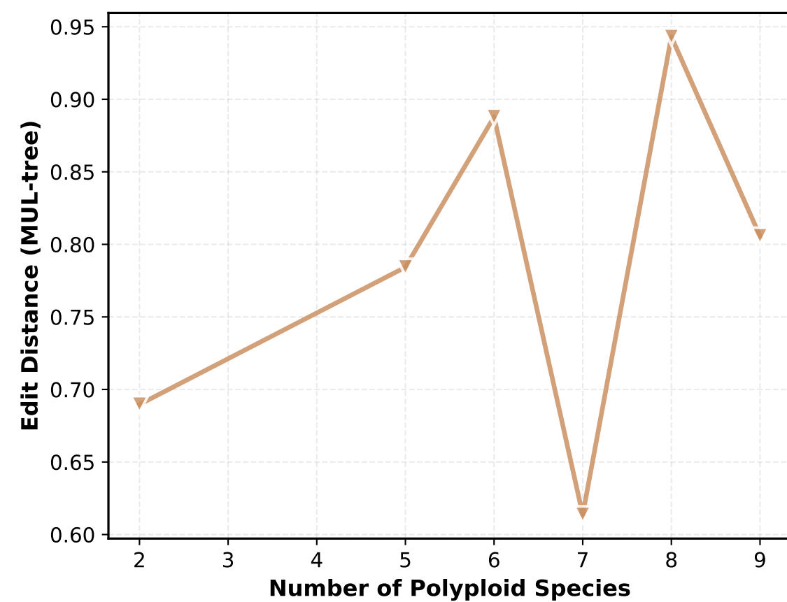
polyphest_p70
