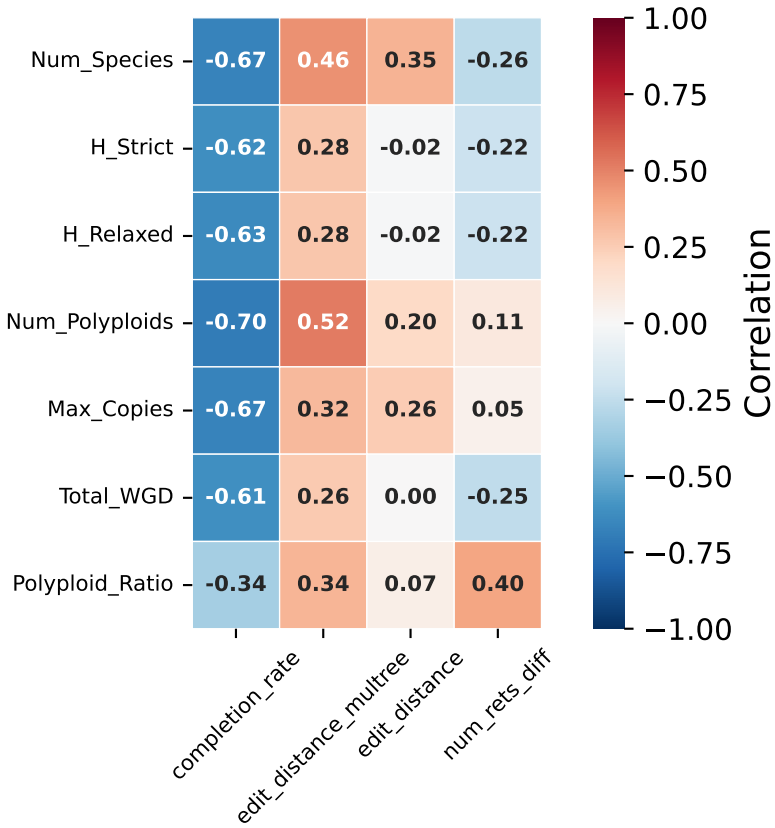
polyphest_p50
