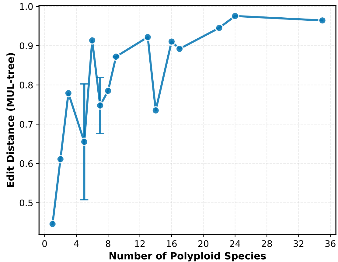
polyphest_p50
