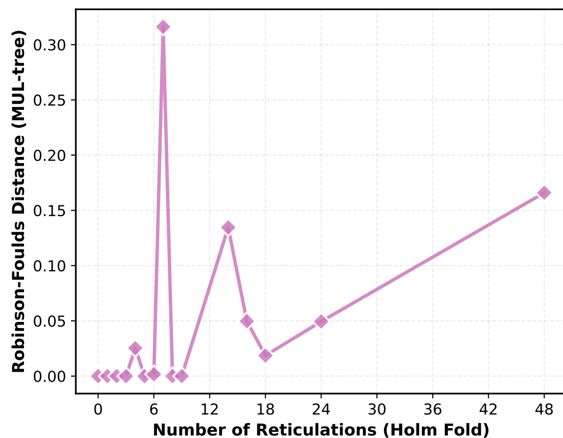
polyphest_p90
