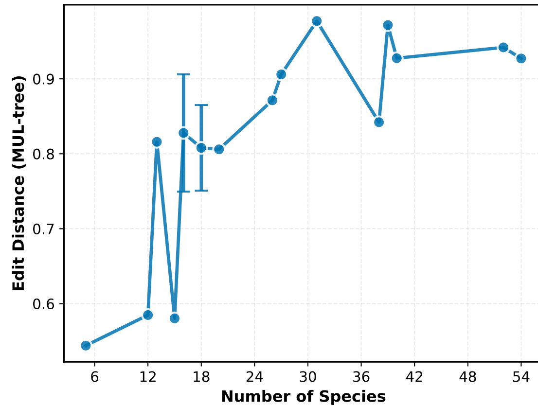
polyphest_p70
