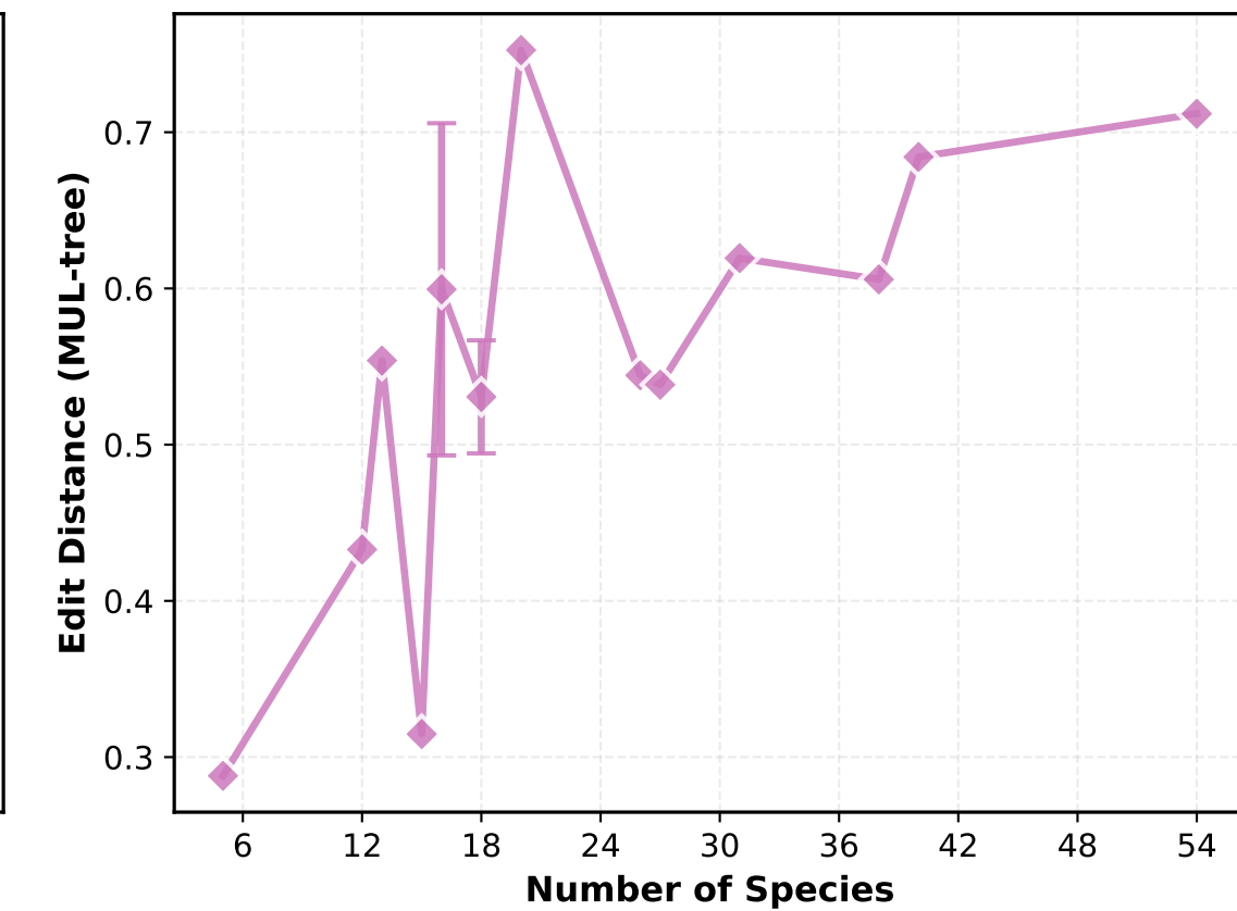
polyphest_p90
