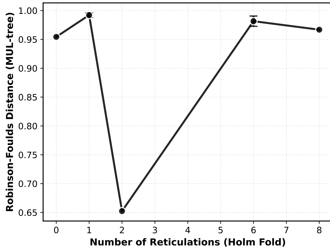
polyphest_p50
