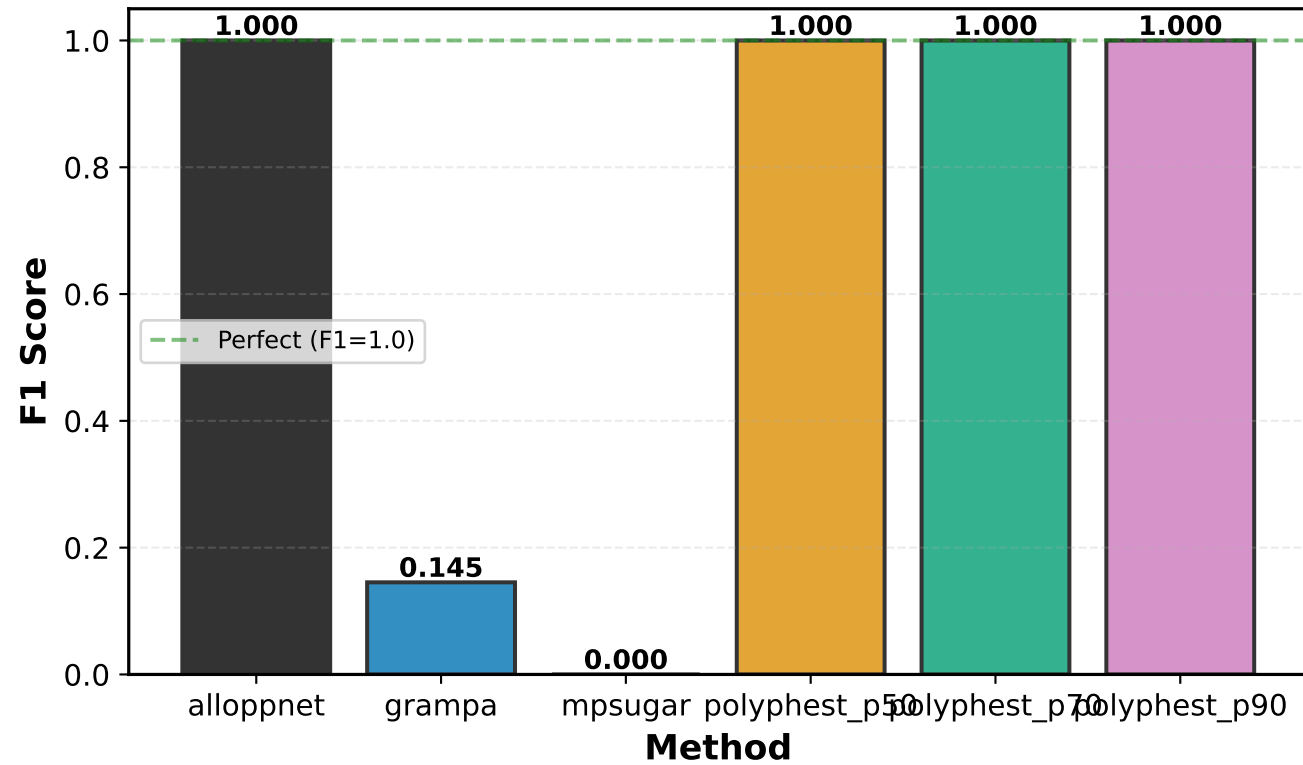
Polyploid Identification F1 Score
