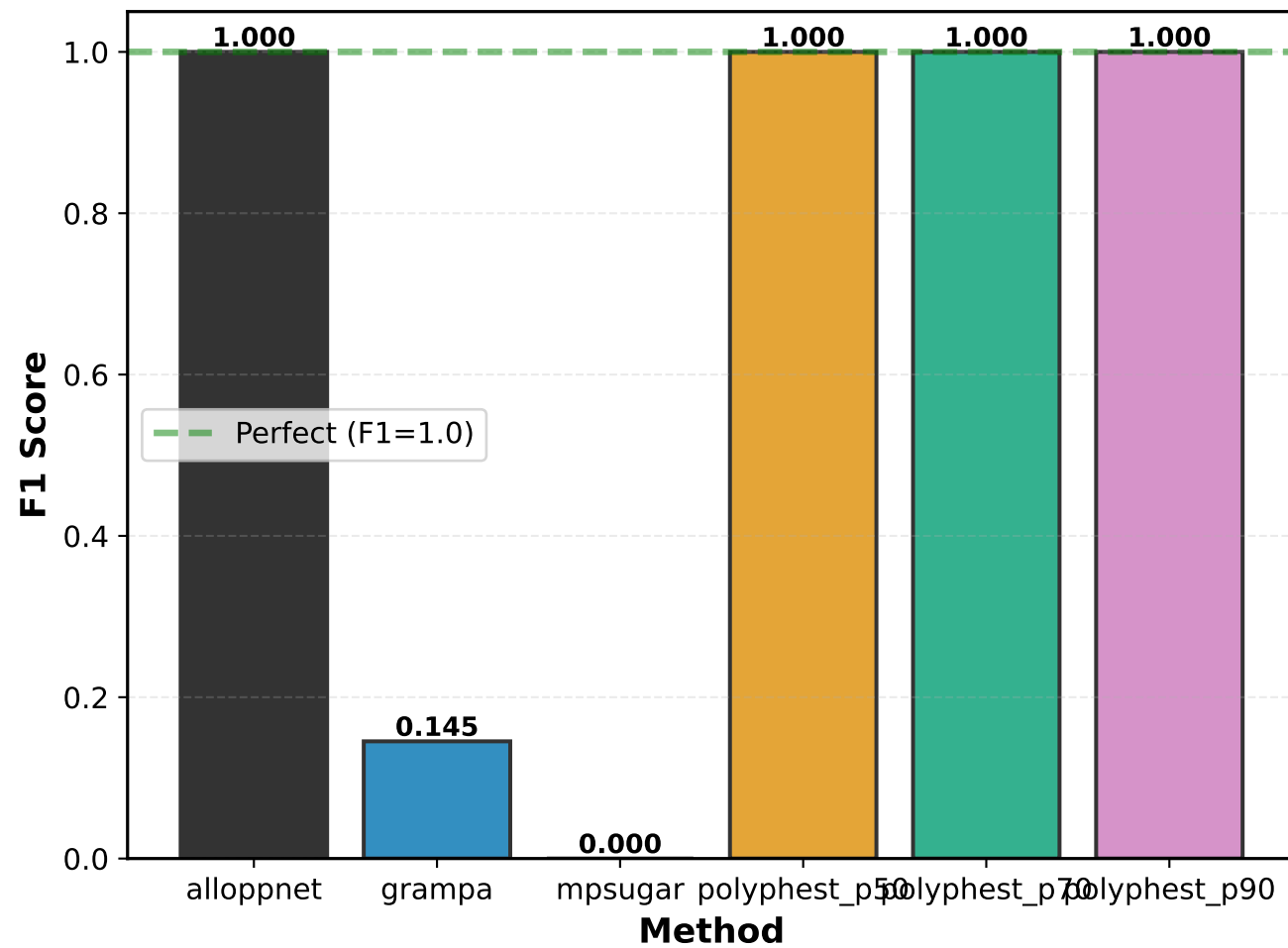
Polyploid Identification F1 Score
