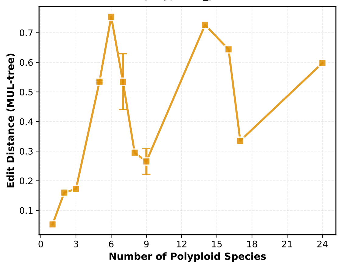
polyphest_p50
