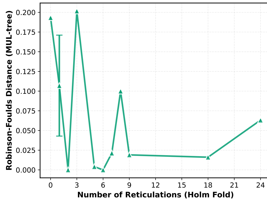
polyphest_p70
