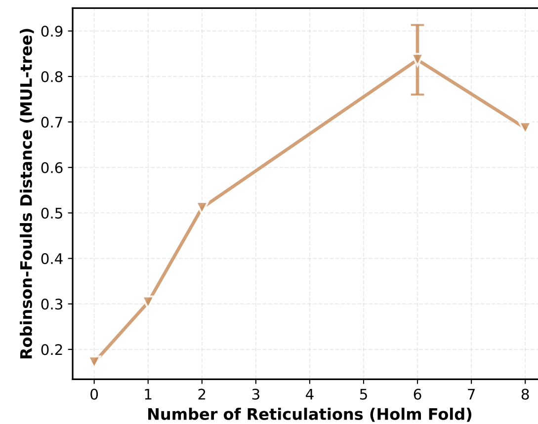
polyphest_p70
