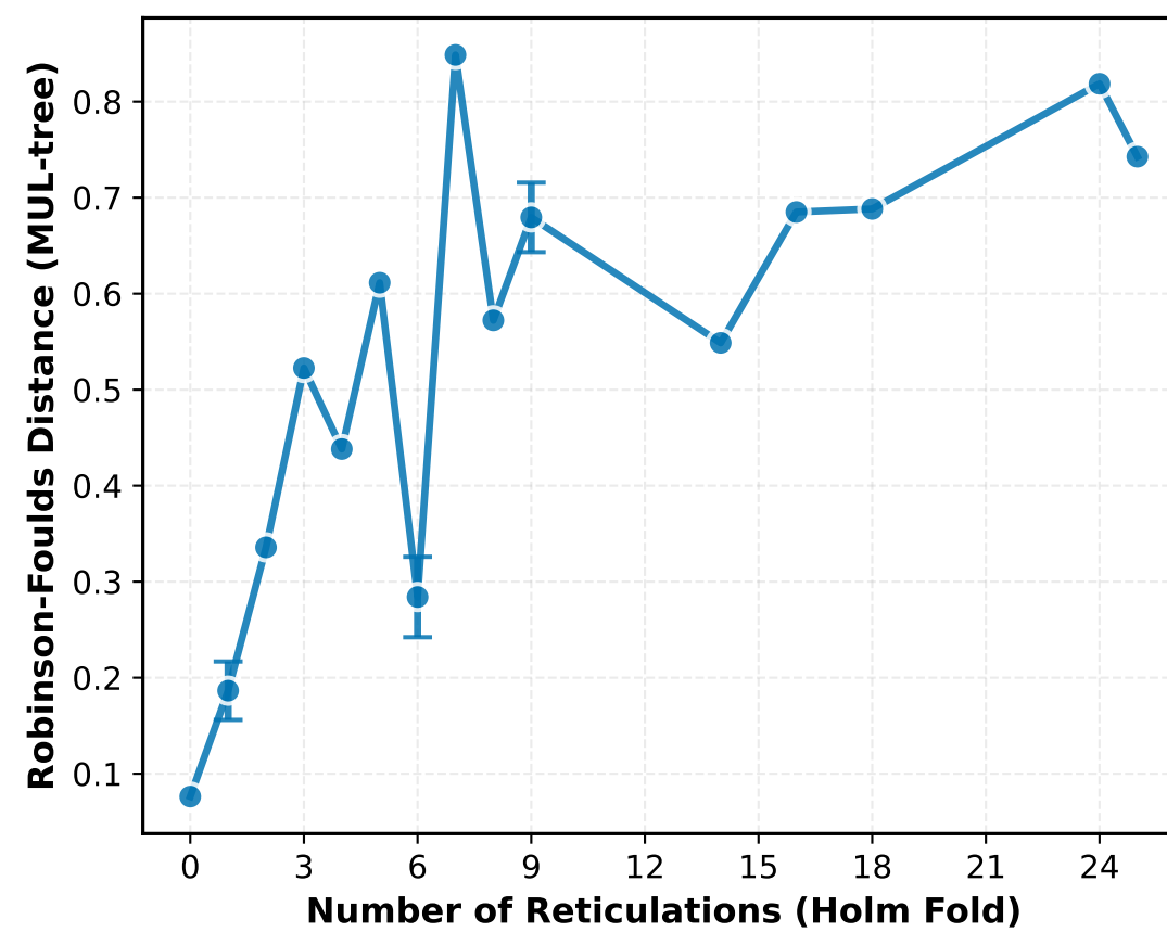
polyphest_p50
