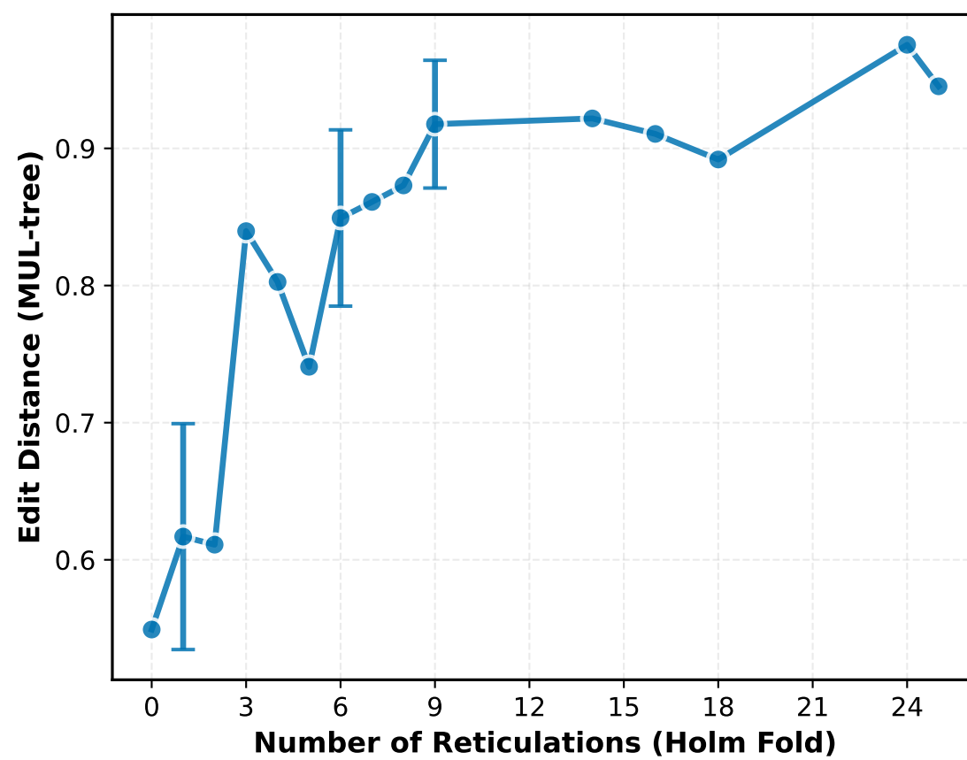
polyphest_p50
