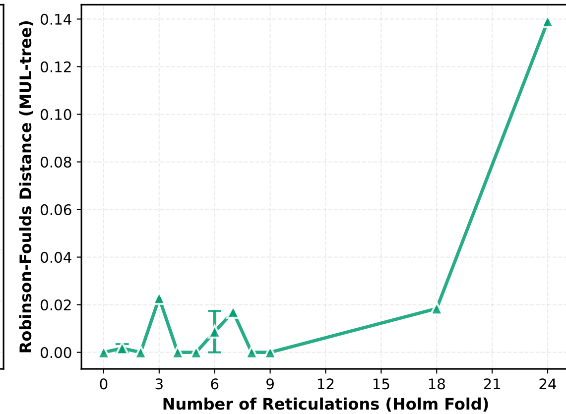
polyphest_p70
