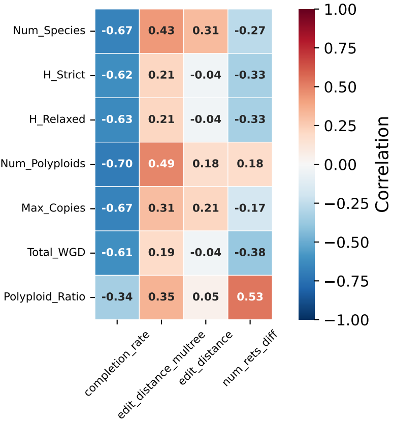
polyphest_p70
