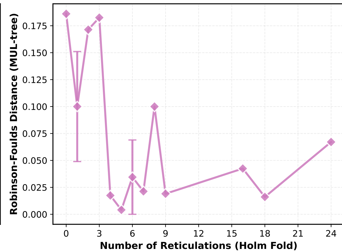
polyphest_p90
