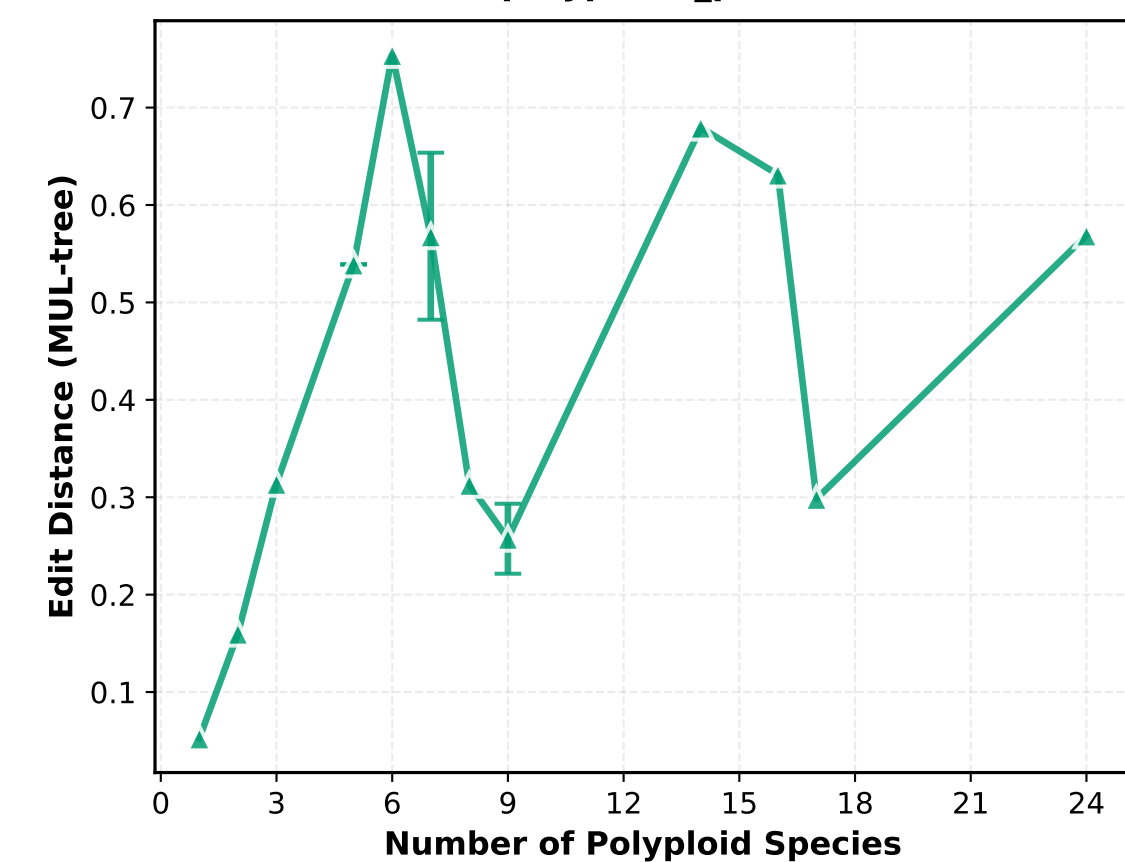
polyphest_p70
