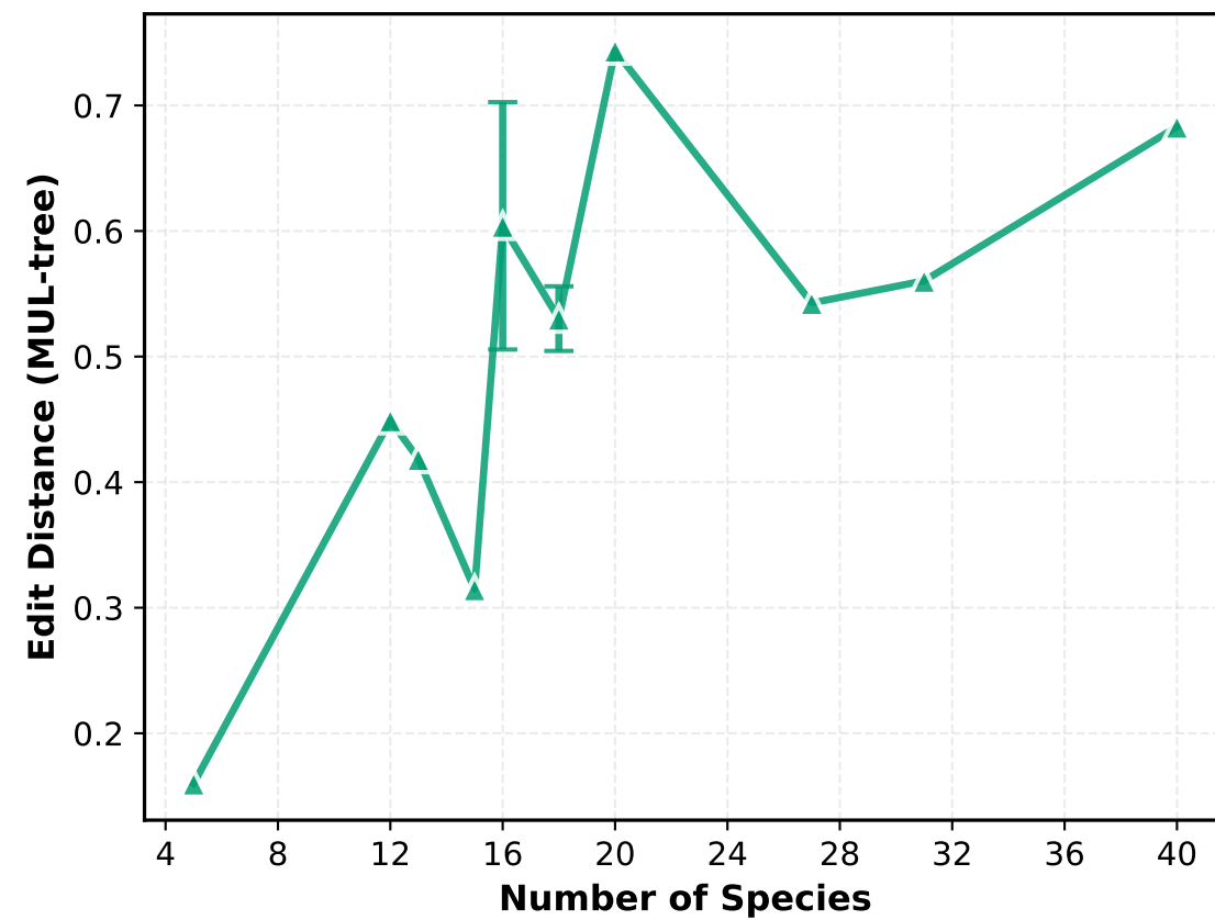
polyphest_p70
