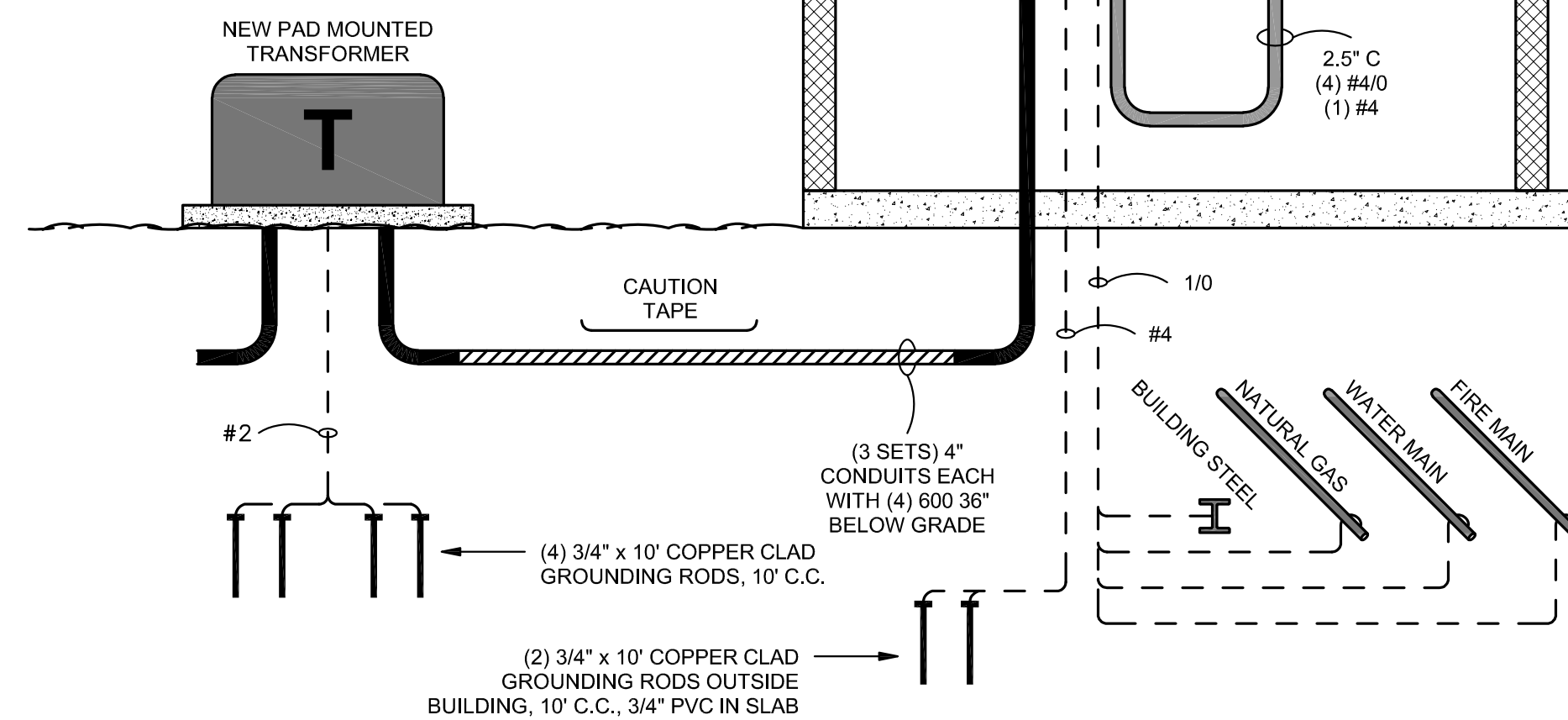
4 E5.1 N.T.S. POWER RISER
