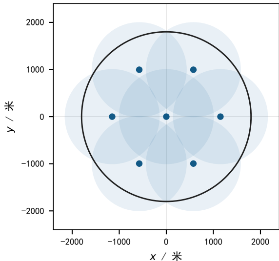
(a) 第三问：七点全向覆盖
