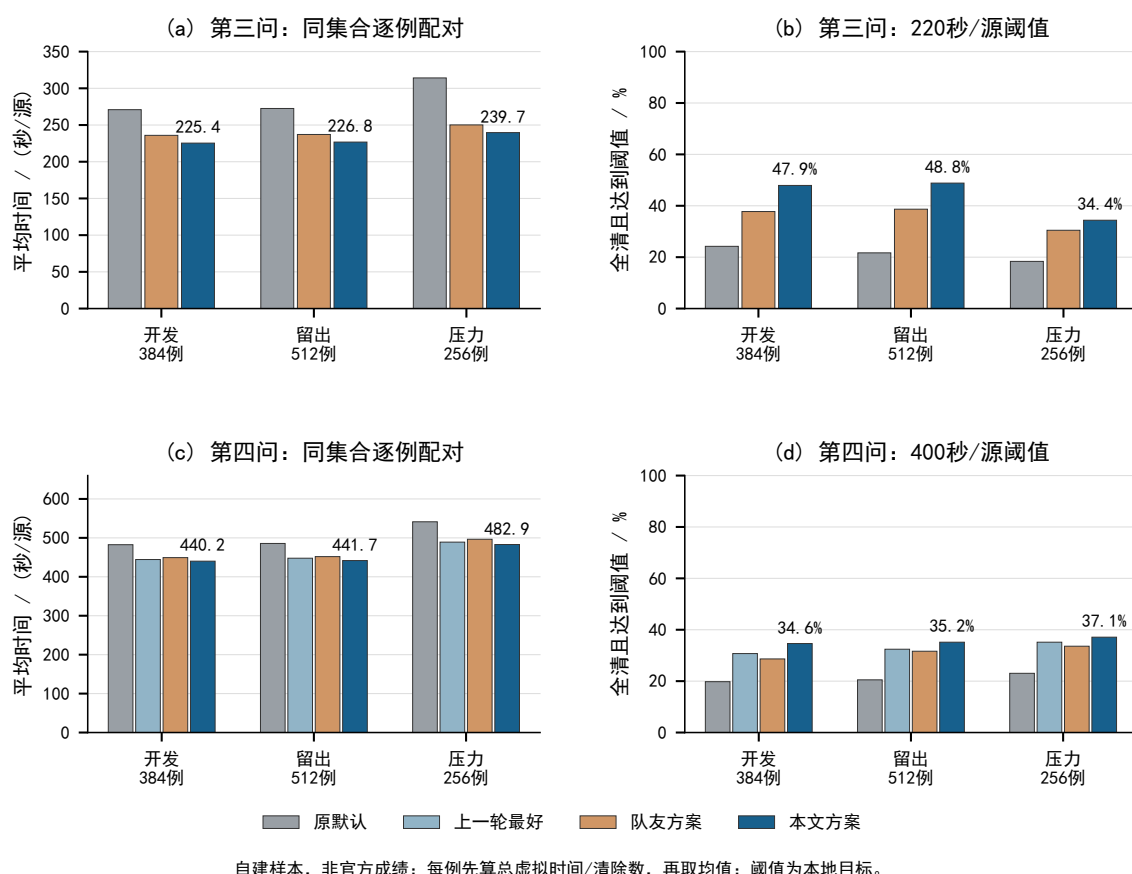
图 5 同一模拟器中的冻结方案配对比较
