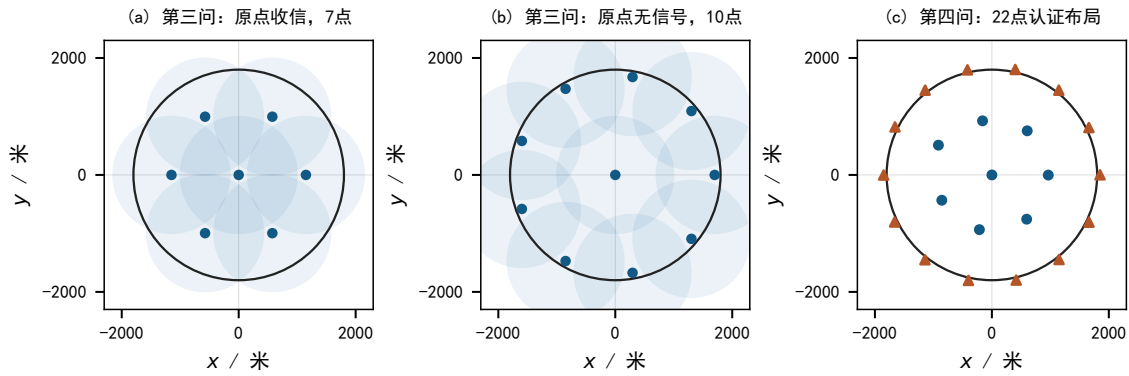
第三问浅色圆盘半径1000米；图示相位不影响覆盖，实际相位按公共状态选择。 第四问蓝点为原点 and 内点、三角为外点；任意朝向覆盖由独立有限几何证书保证。
