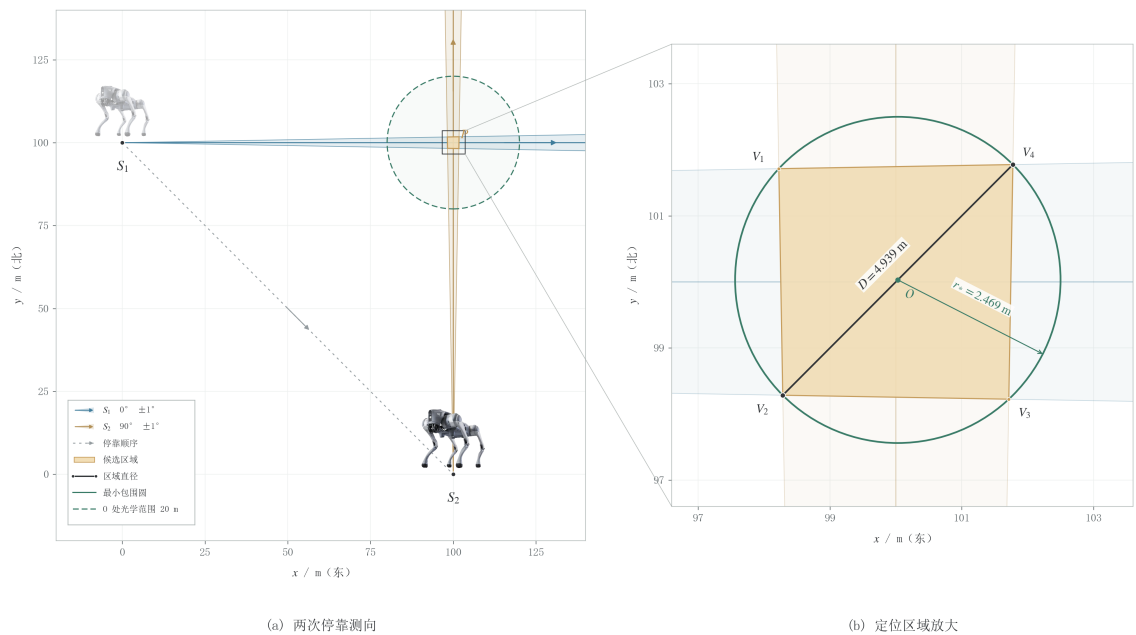
图 1 双站正交交会及定位区域放大图（自建算例）。左图为两次停靠测向及 20 米光学范围，右图为扇区交集；区域直径为 4.939 米，最小覆盖圆半径为 2.469 米。
