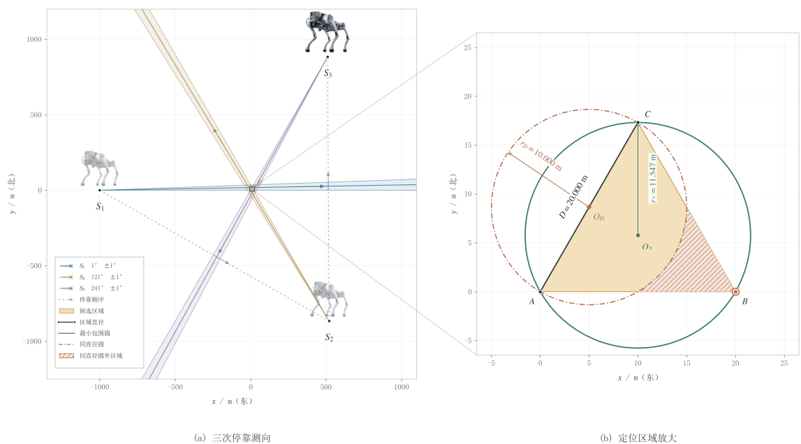
图 2 三站交会形成的等边三角形反例（自建算例，边长 20 米）。左图为三次停靠测向，右图为交集放大图；斜线区未被以 AC 为直径的圆覆盖，最小覆盖圆半径 20/\sqrt{3} \approx 11.547 米大于 D/2 = 10 米。
