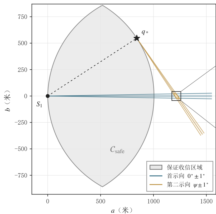
(a) 保证收信的第二检测点
