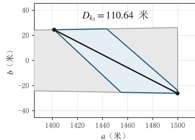
(c) 第 3 组读数单元
