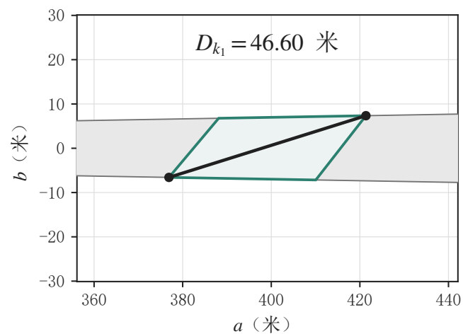
(a) 第 1 组读数单元
