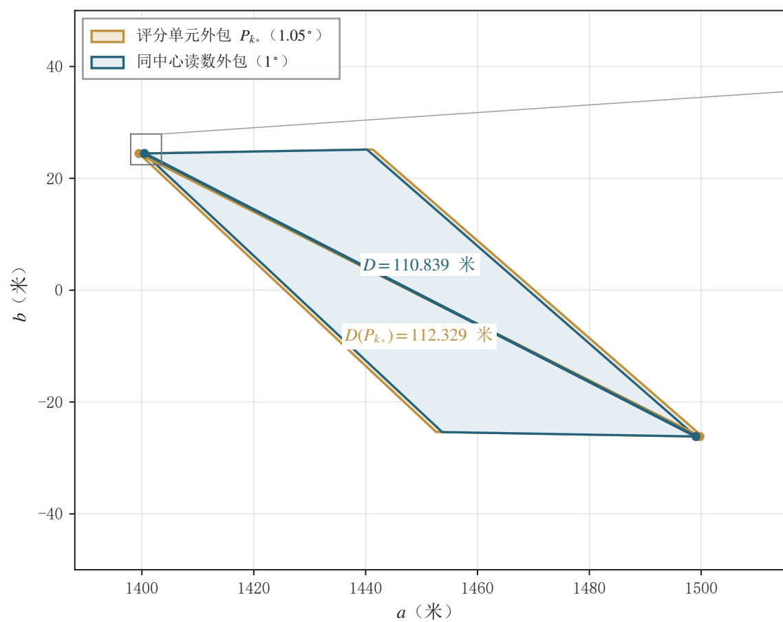
(a) 固定读数 \psi = 317.9^\circ
