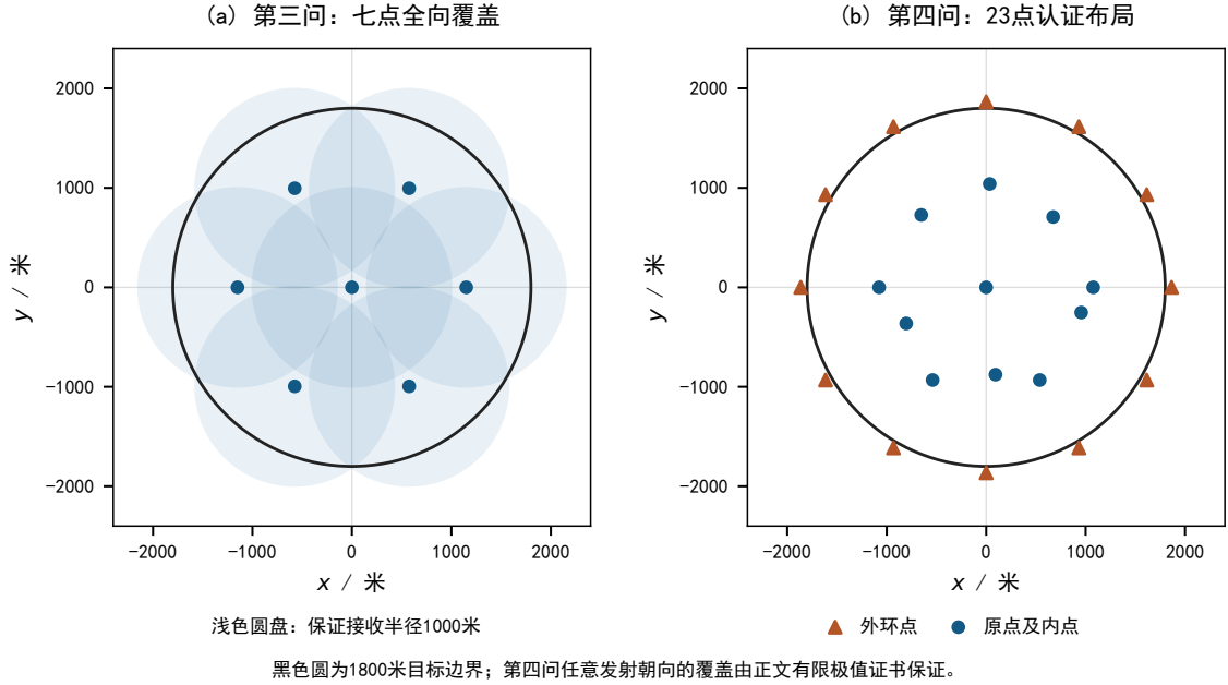
图 9 第三问全向覆盖与第四问认证检测布局
