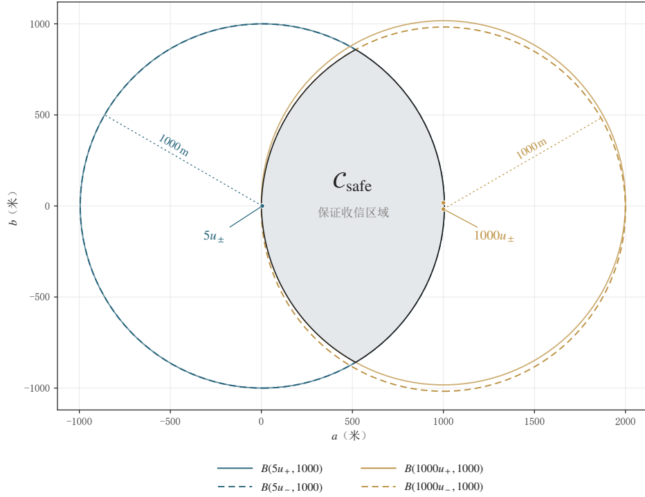
图 4 四圆盘交集构成的保证收信区域 C_{\text{safe}}
