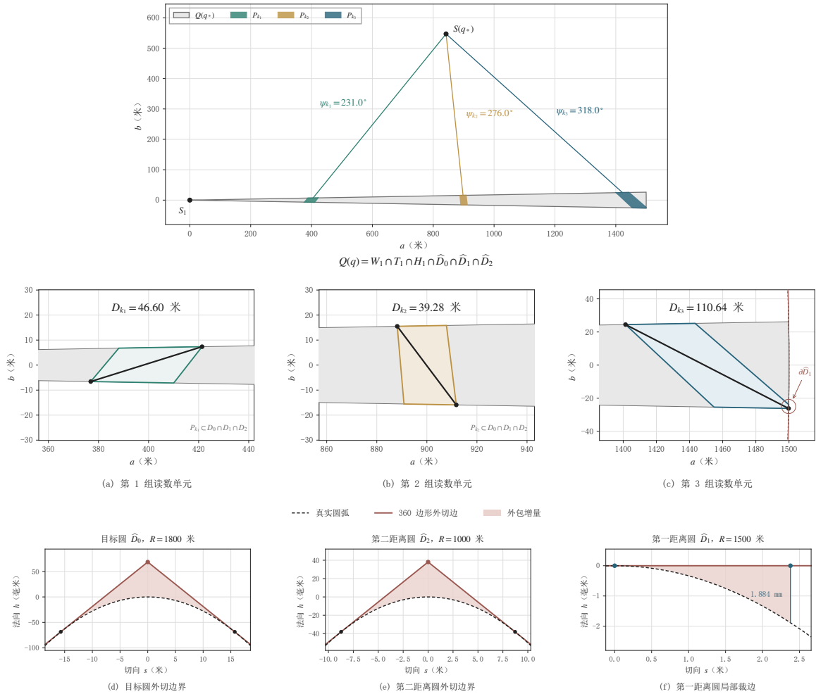
图 6 同一候选点下的读数单元、几何外包及圆边界近似
