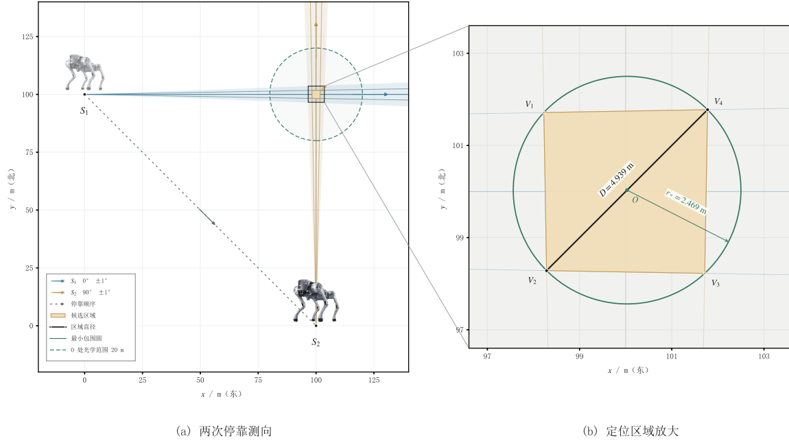
图 2 双站正交测向及交会区域（自建算例）。左图为检测点与示向扇区，右图为交会区域及其直径、最小覆盖圆的放大图。
