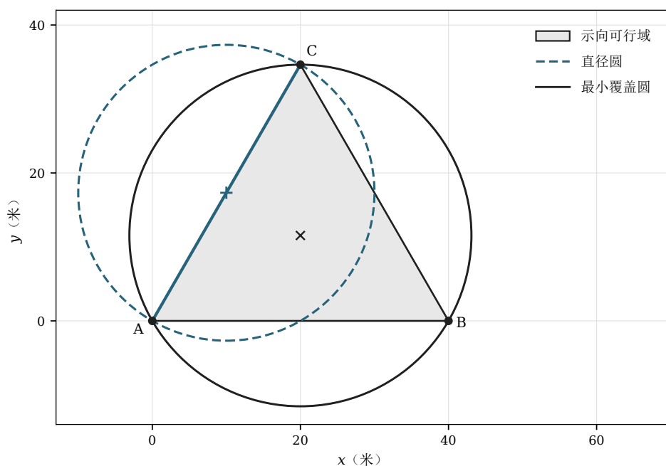
图3 直径圆不能覆盖定位区域的反例（自建算例，边长40米）。以AC为直径的圆未覆盖顶点B；最小覆盖圆半径为 40/\sqrt{3} \approx 23.094 米，大于20米。
