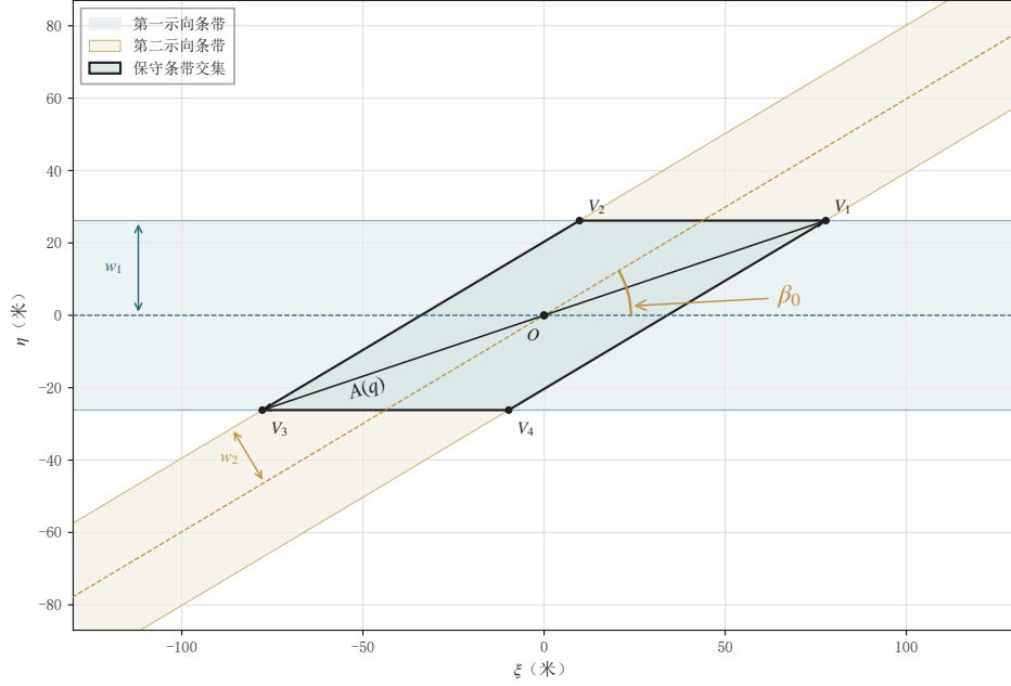
图 5 评分一的条带交集与解析直径：夹角取下界 \beta_0 ，双向箭头沿长对角线标示 A(q)
