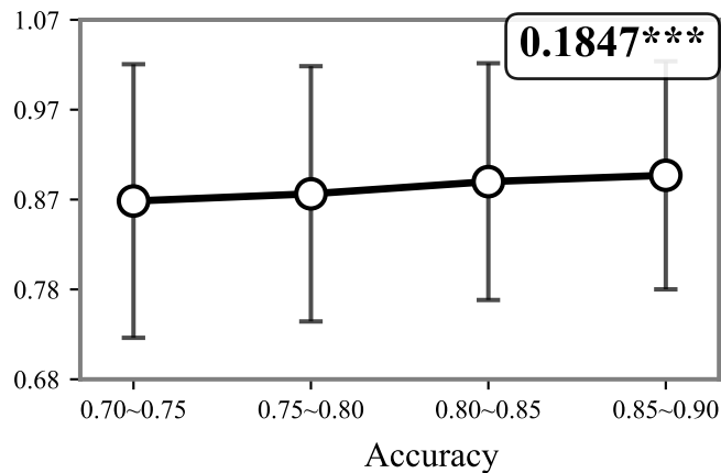
LIME
