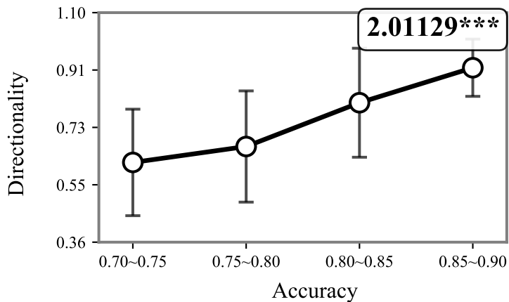
SHAP
